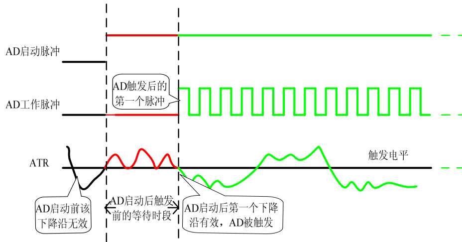
5.3 下降沿触发图例
