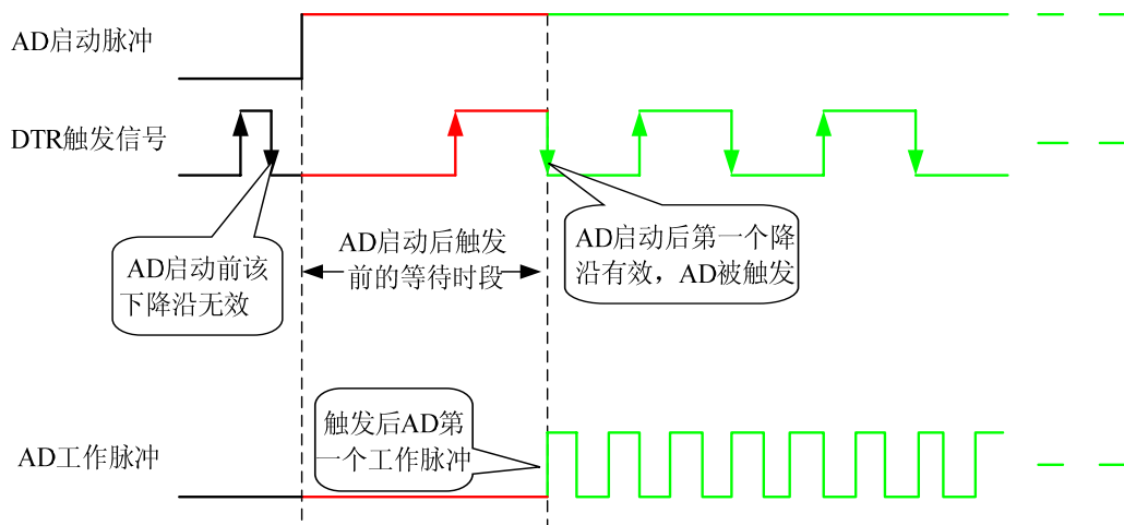
5.4 下降沿触发图例
