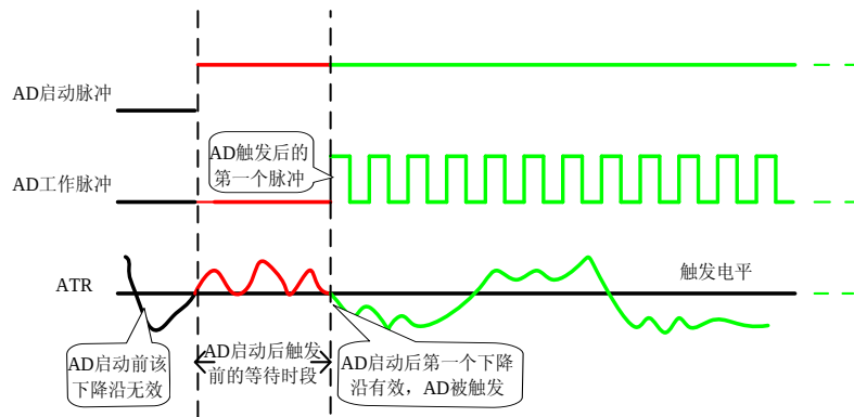
5.3 下降沿触发图例
