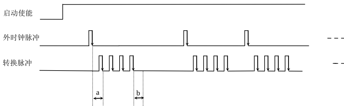
图 6.11 不固定频率外时钟模式下的分组
