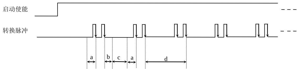
图 6.8 内时钟模式下组循环次数为“1”的分组采集
