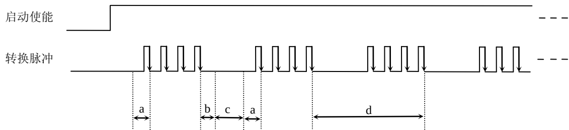
图 6.9 内时钟模式下组循环次数为“2”的分组采集
