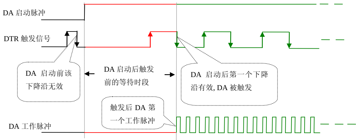
图 6.16 下降沿触发图例
