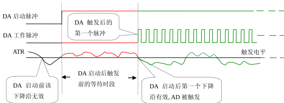
图 6.14 下降沿触发图例，上升沿同理
