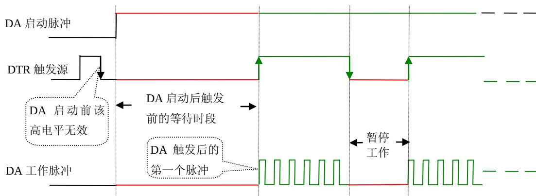
图 6.17 高电平触发图例
