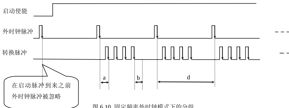
图 6.10 固定频率外时钟模式下的分组
