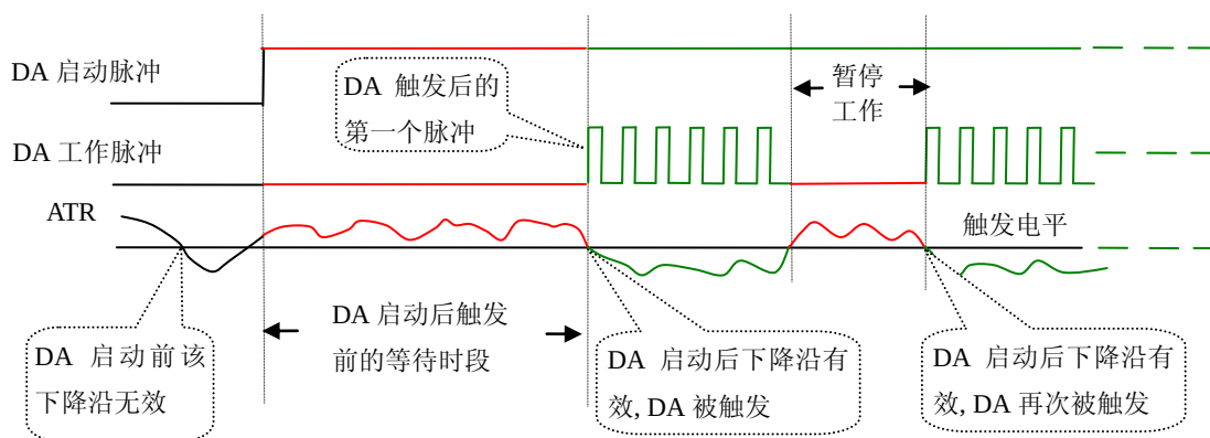
图 6.15 低电平触发
