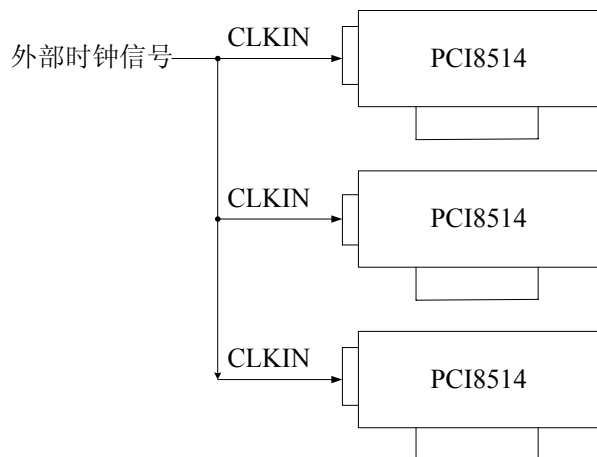
外时钟同步采集的连接方法
