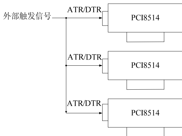
外触发同步采集的连接方法
