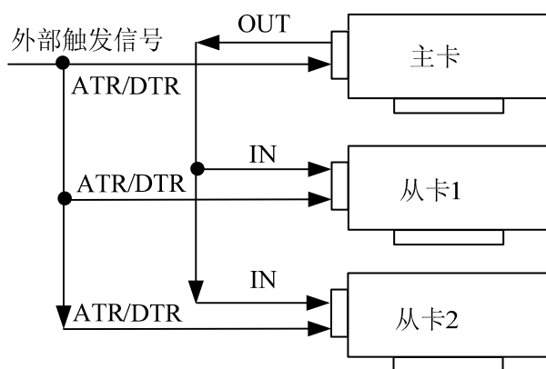
主从卡 级联 采用共同的外触发连接方法
