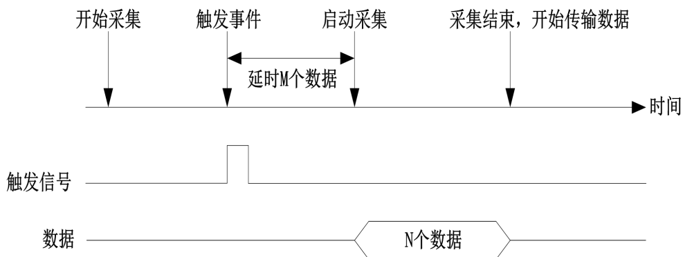
图 4-7-4 硬件延时触发
