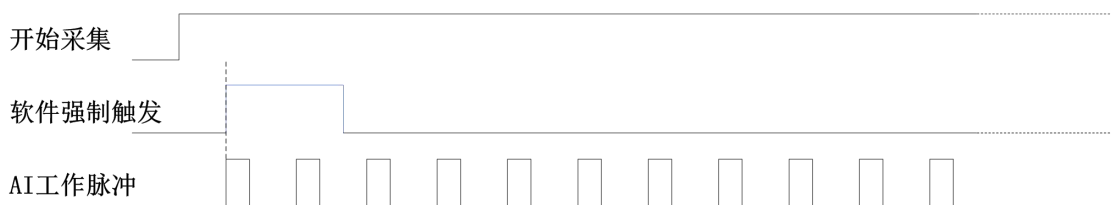
图 4-8-3 AI 软件强制触发
