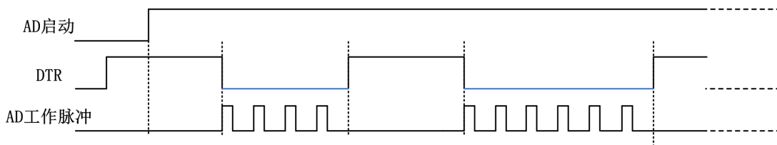
图 4-7-6 暂停触发—高电平暂停
