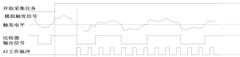
图4-8-6 模拟边沿触发--下降沿触发
