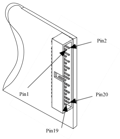
图 3-2-2 RTSI 的 Pinout 图
