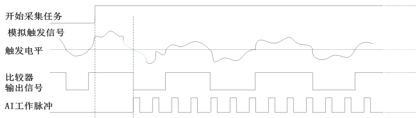
图4-8-8 模拟窗触发--入窗
