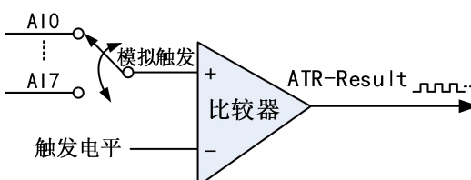
图4-8-7 比较器
