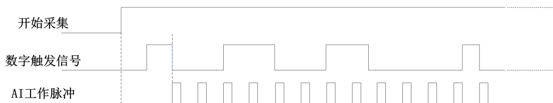
图4-8-10 数字边沿触发--下降沿触发
