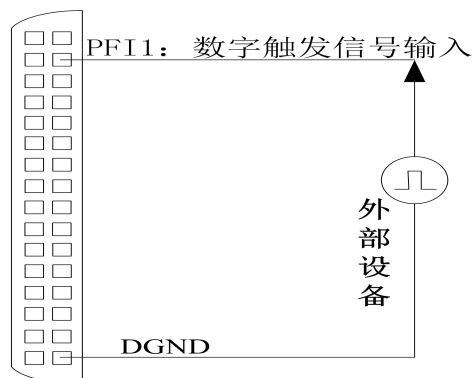
图4-8-9 数字触发连接方法
