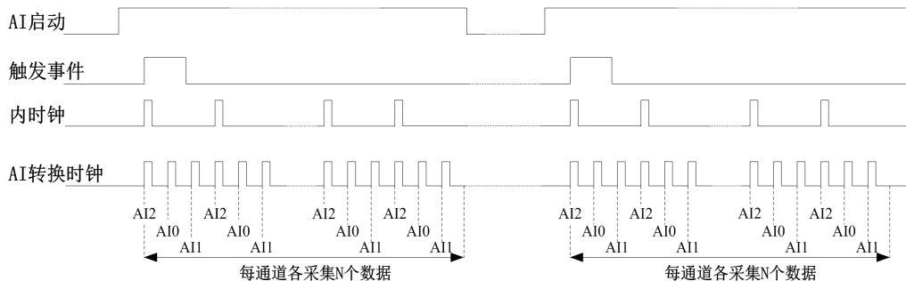
图4-6-2 有限点采样
