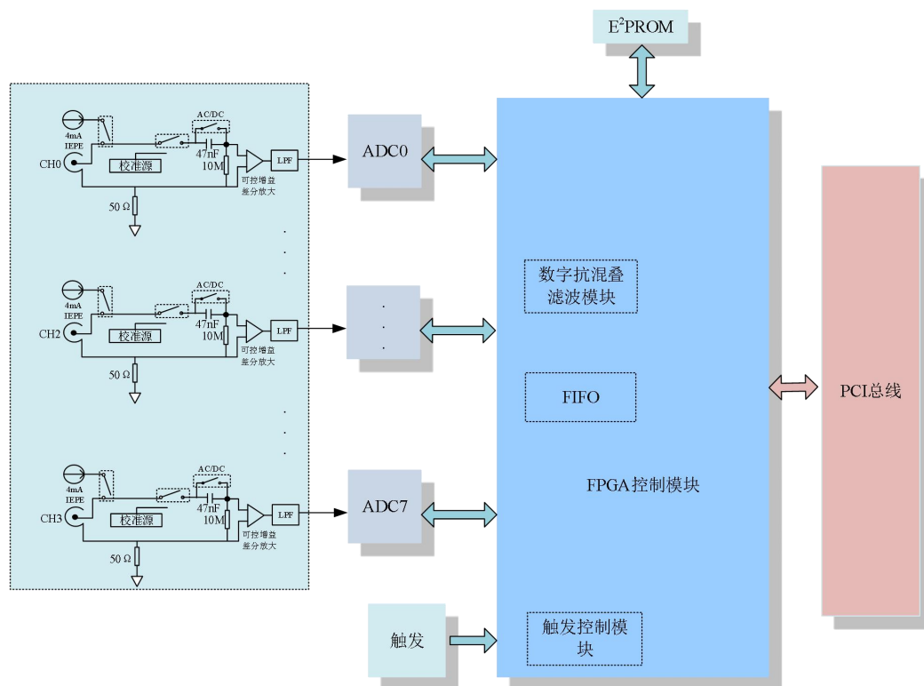
图 2.2.1 PCI8814 系统框图
