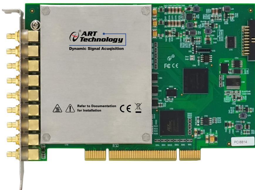
图 3-1-1 PCI8814 外形图
