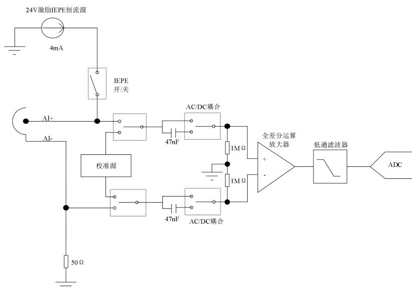
图 4.1.1 模拟输入功能框图
