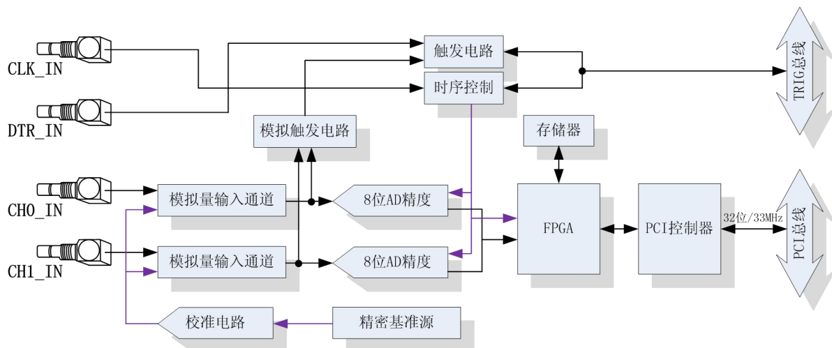
图 2-2-1 PCI8520B 系统框图
