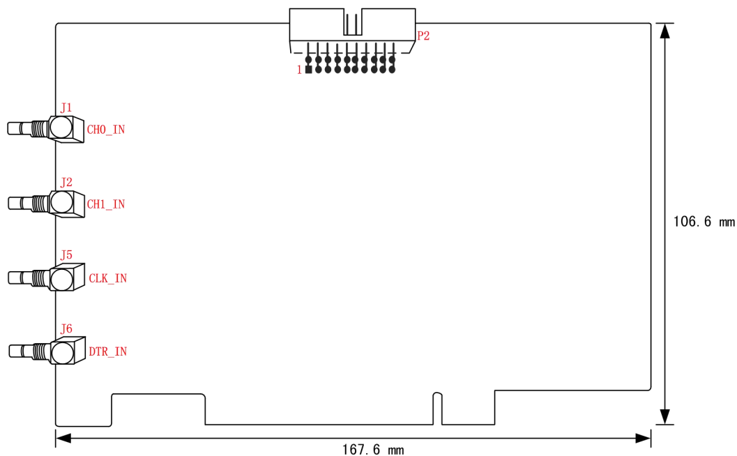
图 3-1-1 PCI8520B 板卡尺寸图
