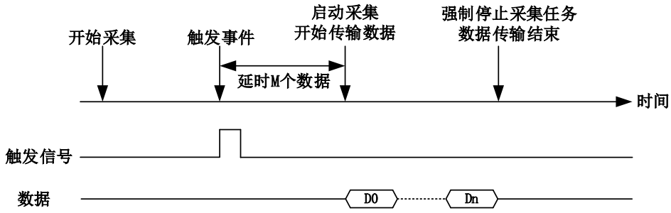
图4-9-1-2 硬件延时触发模式下连续采样
