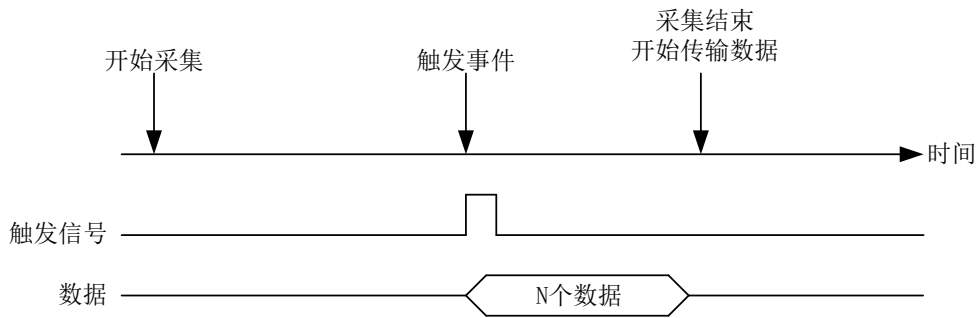
图 4-9-2-3 后触发
