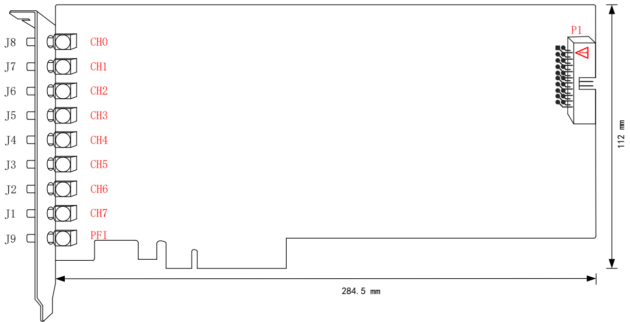
图 3-2-1 PCIe8582/8584/8586 板卡尺寸图
