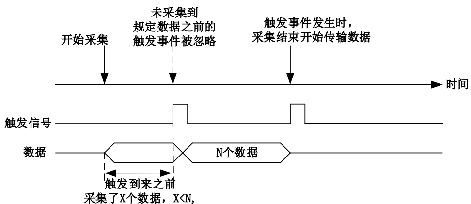
图 4-9-2-5 预触发--采集数据小于 N
