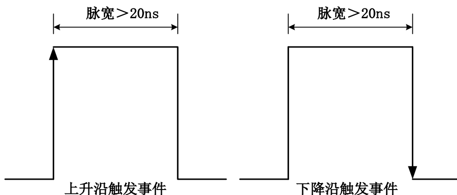
图 4-8-8 脉宽最小值图
