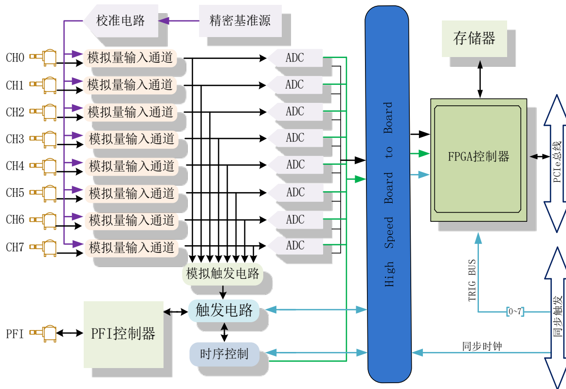
图 3-1-1 PCIe8582/8584/8586 系统框图
