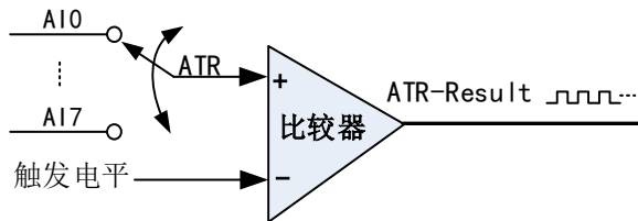
图 4-8-5 比较器
