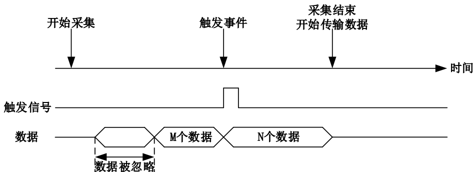
图 4-9-2-2 中间触发
