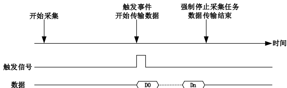
图4-9-1-1 后触发模式下连续采样
