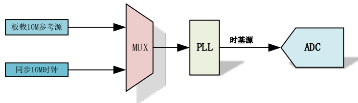
图 4-7-1 时基源框图
