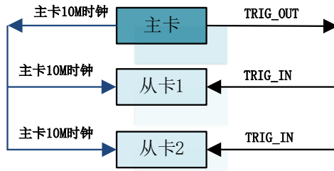
图 4-10-1 主从卡级联
