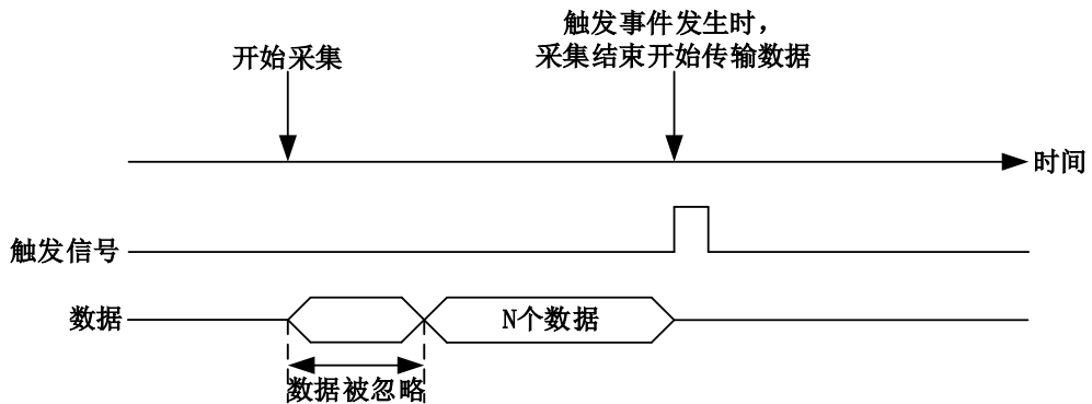
图 4-9-2-4 预触发
