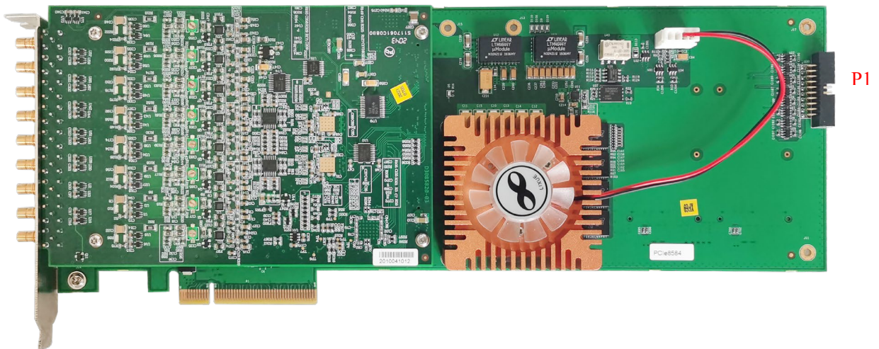
图 3-3-1 PCIe8582/8584/8586 产品外观图
