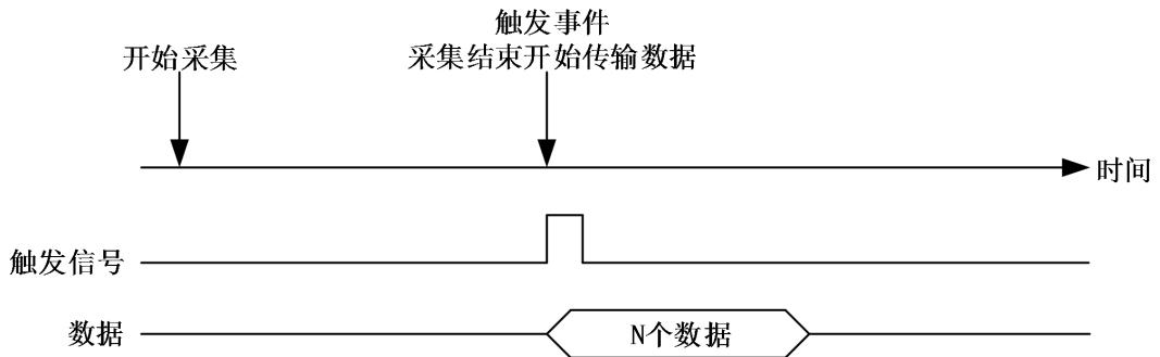
图 4-9-2-3 后触发
