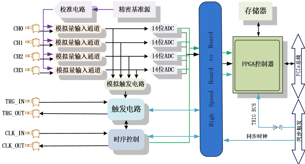
图 3-1-1 PCIe8504/8514 系统框图
