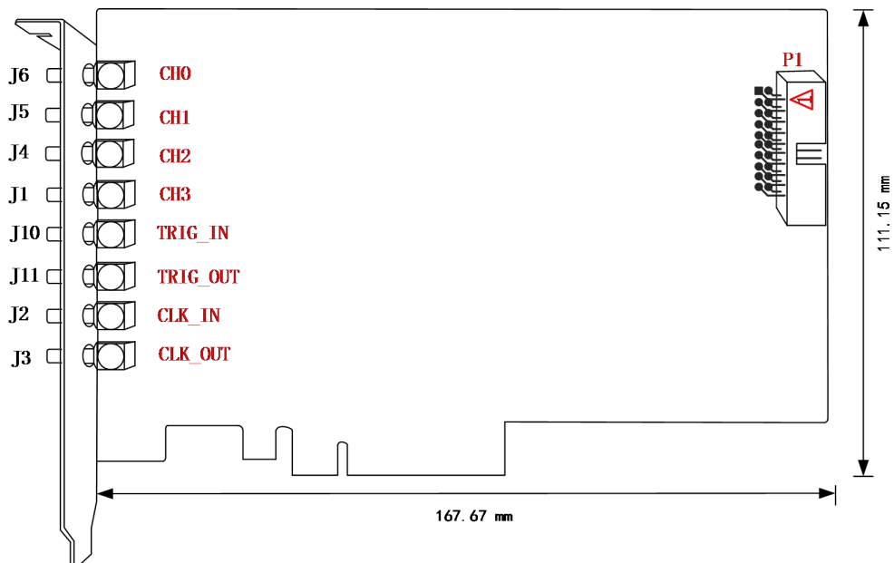
图 3-2-1 PCIe8504/8514 板卡尺寸图
