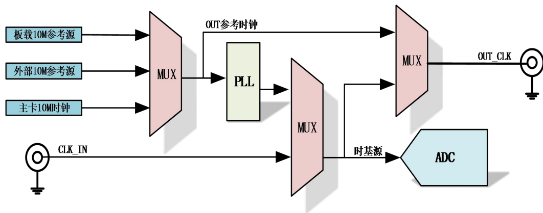
图 4-7-1 时基源框图
