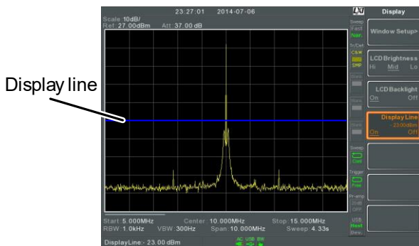
-50dBm 显示线
