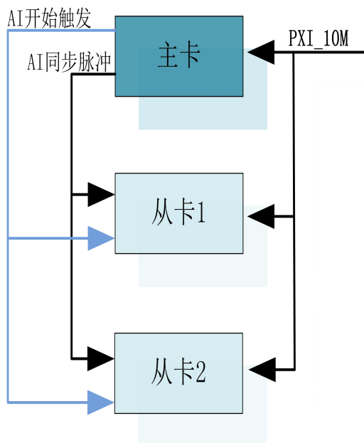
图 4-9-1 主从卡级联
