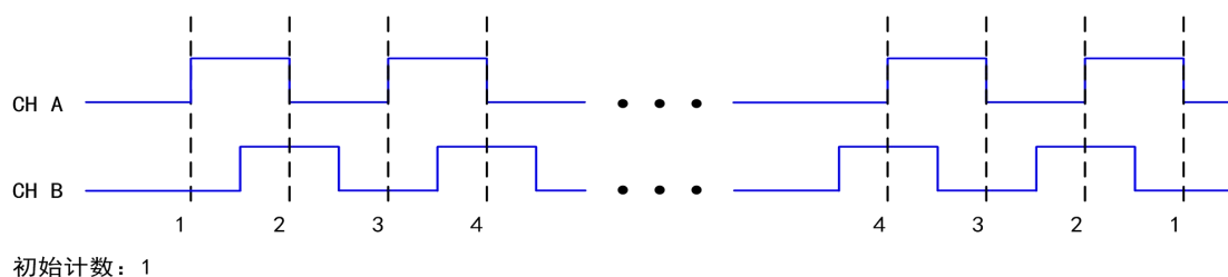
图 5-7-2 X2 编码
