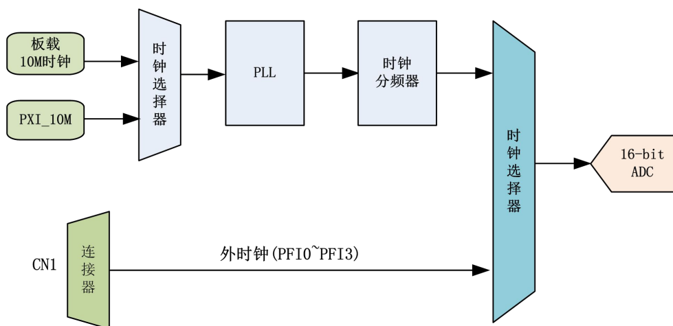
图 4-6-1 AI 时钟结构框图
