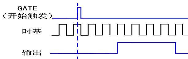
图 5-8-2 具有启动触发的单脉冲生成
