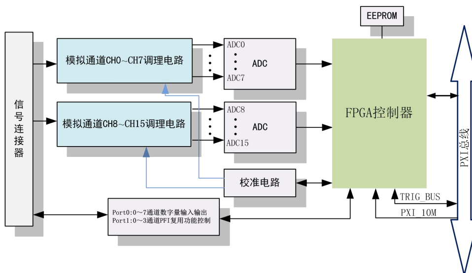
图 2-2-1 PXI9009 系统框图
