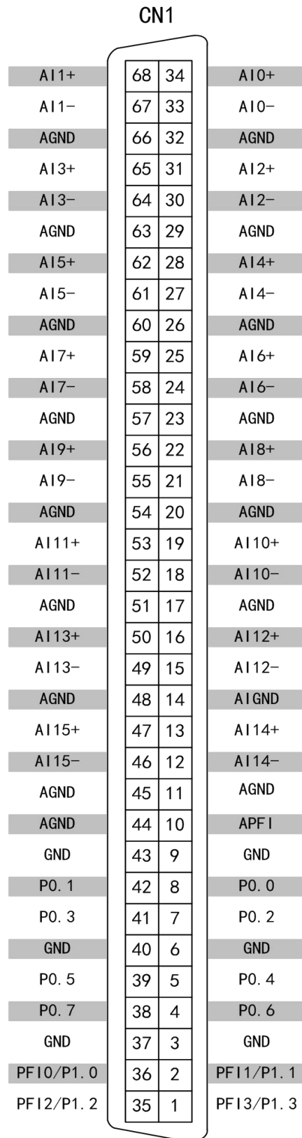
图 3-3-1 PXI9009 管脚定义图
