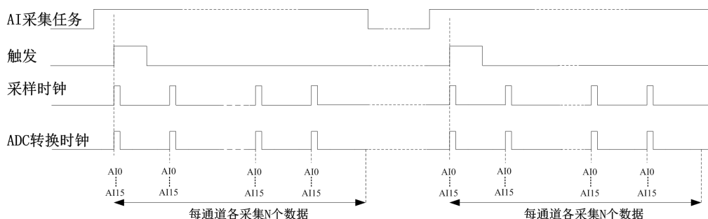
图 4-7-2 有限点采样
