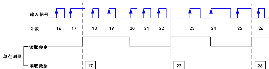
图 5-1-1 边沿加计数上升沿有效示意图
