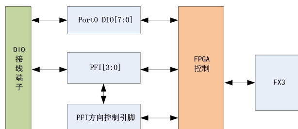
图6-1-1 DIO功能框图
