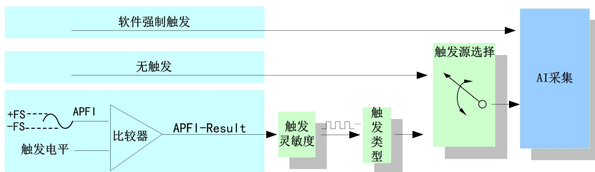
图 7-1-2 模拟触发源选择
