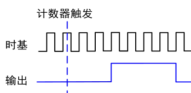
图 5-8-1 单脉冲生成
