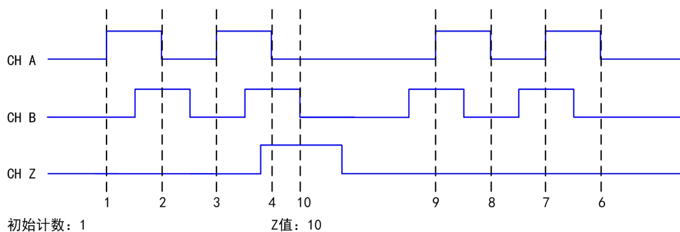
图 5-7-6 Z 索引
