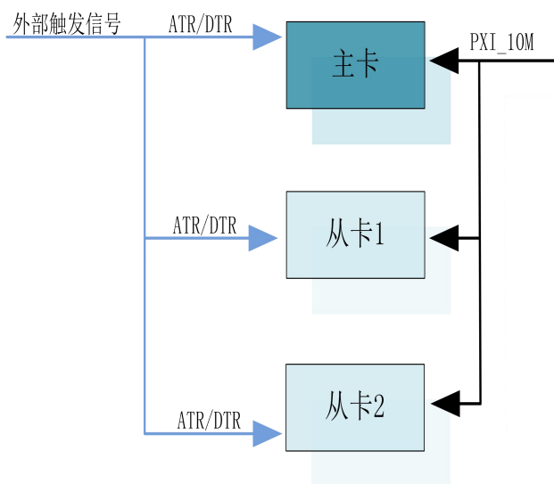
图 4-9-2 共同的外触发信号
