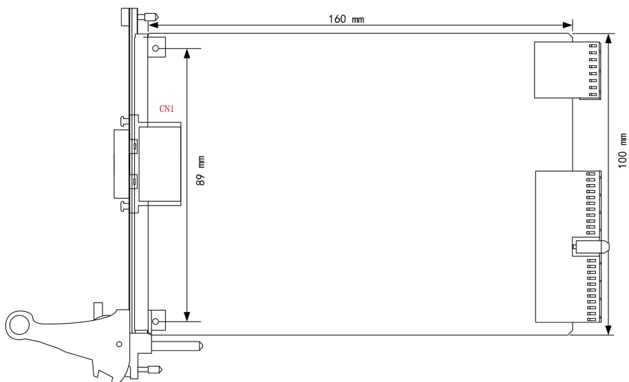
图 3-2-1 PXI9009 板卡尺寸图
