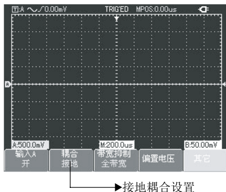
图2-8 接地方式下屏幕显示
