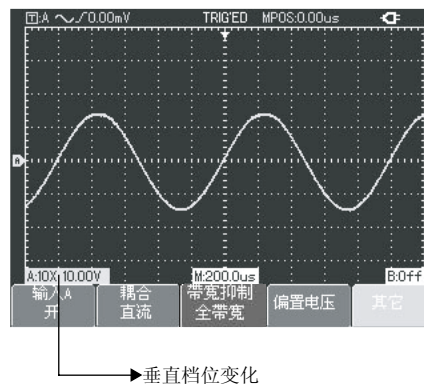
图2-12 垂直单位的变化
