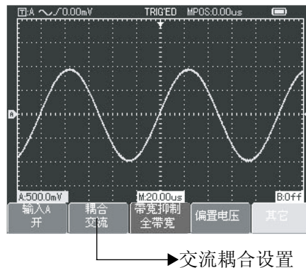
图2-7 只显示被测的交流信号
