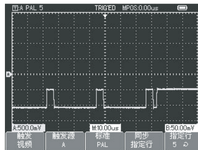
图3-9 视频指定行触发
