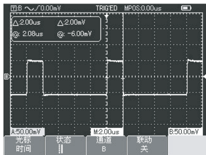
图3-6 光标测量脉冲宽度
