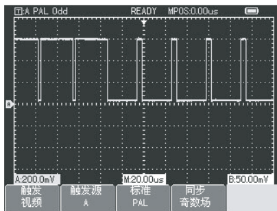
图2-18视频触发： 场同步
