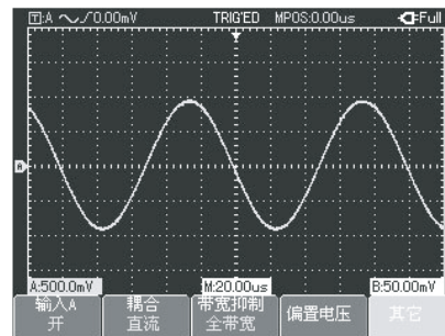
图2-15通道极性设置（反相）
