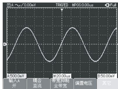
图2-14通道极性设置（正常）
