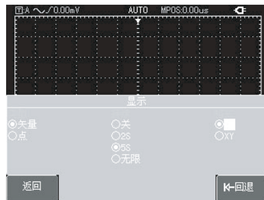
图2-5使用拨盘进行“格式”菜单操作
