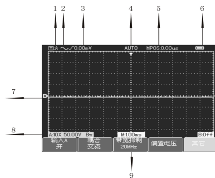
图1-2 显示界面说明图
