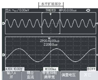
图2-28 视窗扩展下的屏幕显示
