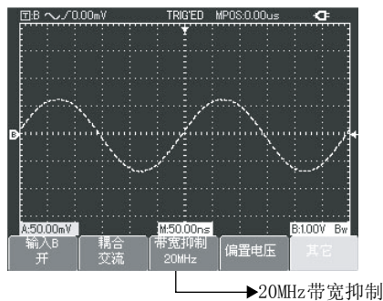
图2-10 20MHz带宽限制
