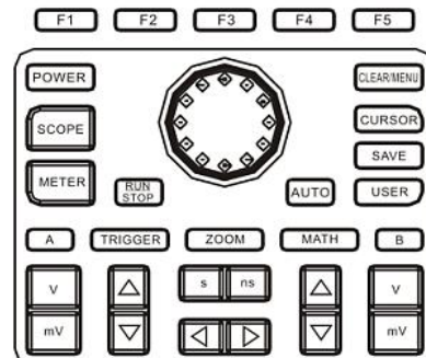
图1-7 示波表操作面板
