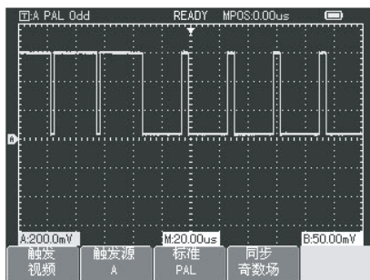
图3-8 视频奇数场触发
