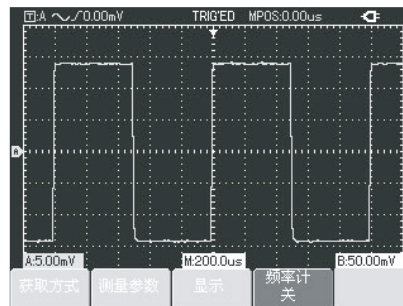
图3-5 信号噪声被抑制
