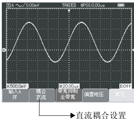
图2-6 被测信号的直流分量和交流信号同时显示
