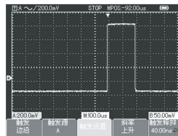
图3-3 单次信号触发
