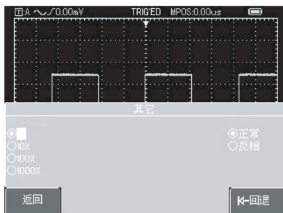
图1-4 探头倍率调整
