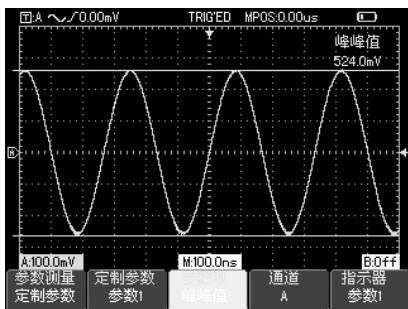
图2-22 指定参数测量
