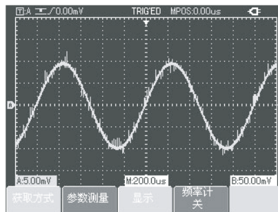
图2-20 未做平均前的波形
