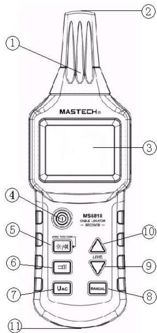
接收机平面图
