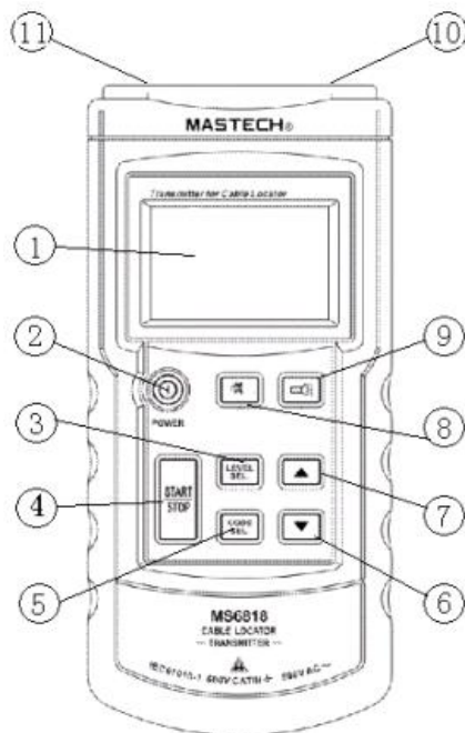
发射机平面图
