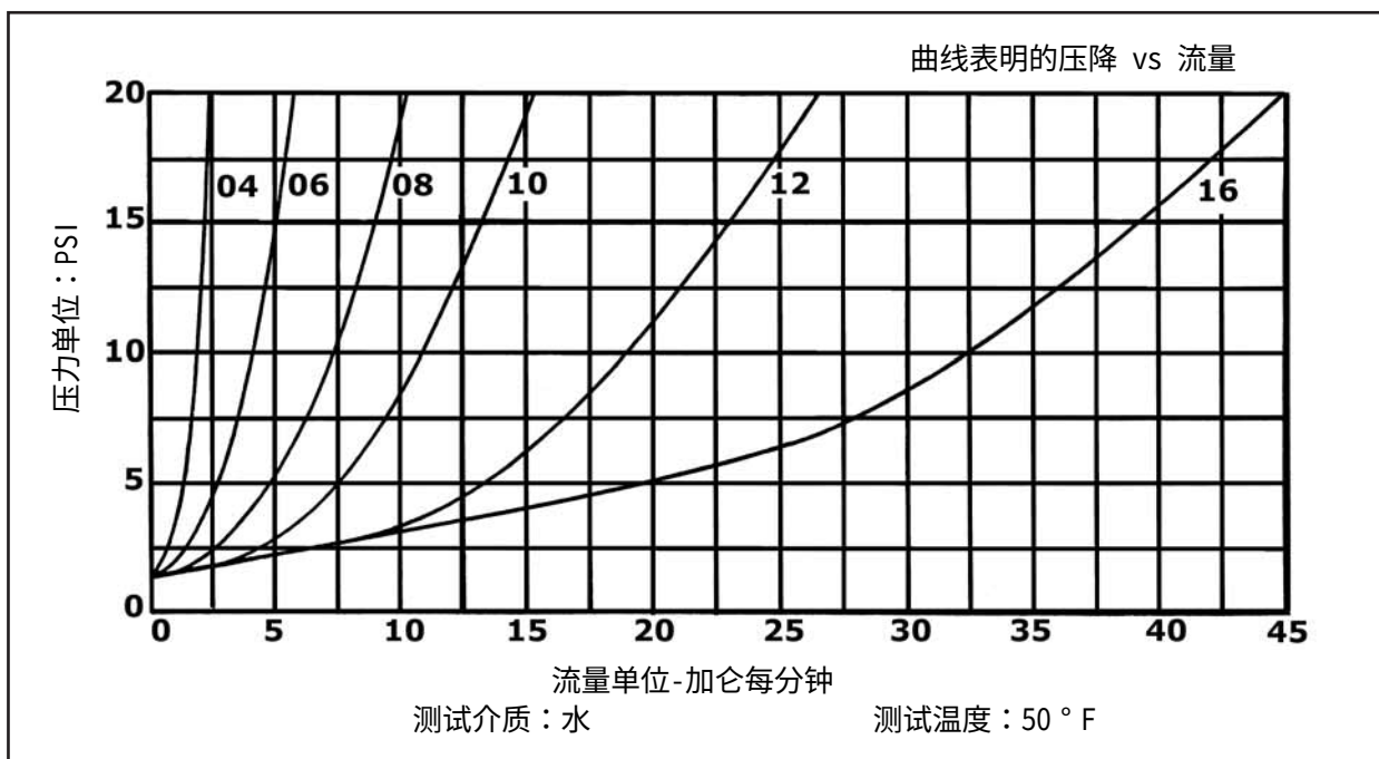
流量曲线图：1/8" - 1"规格
