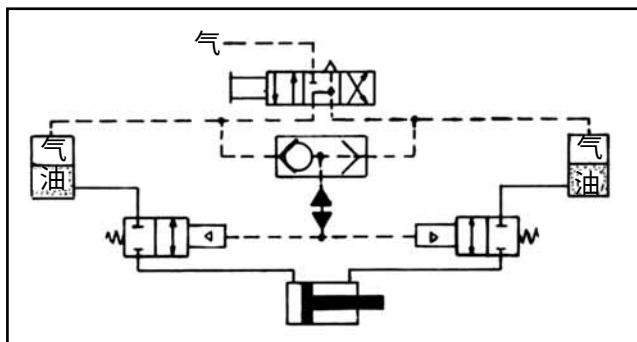
气动先导式控制回路
