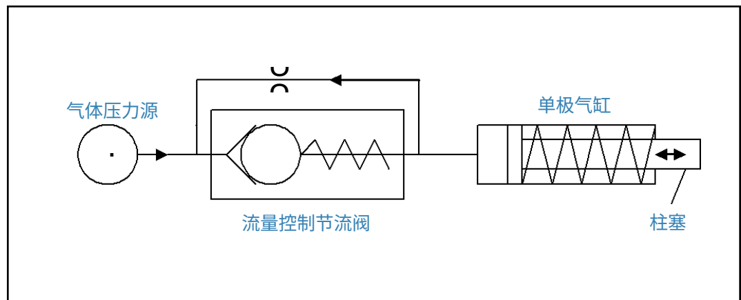
节流阀的流量控制应用图例
