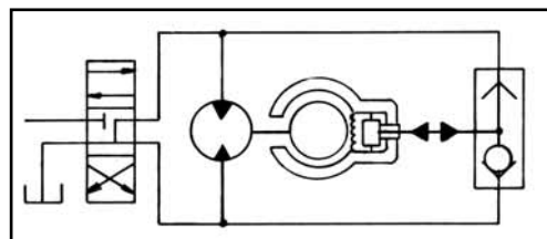
刹车制动回路
