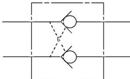
ANSI标准符号
