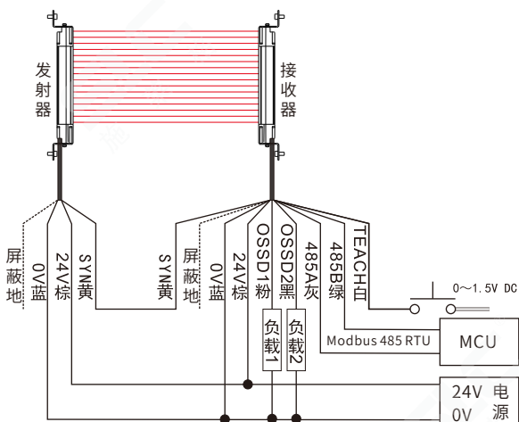
电流模拟量输出接线图
