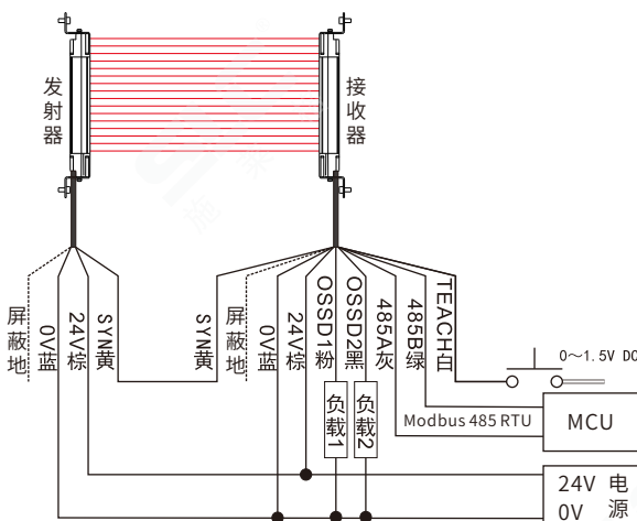
电压模拟量输出接线图
