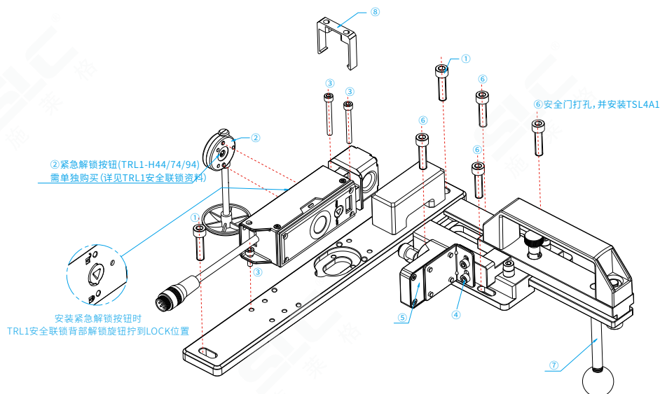
TSL4配TRL1系列安全联锁安装图
