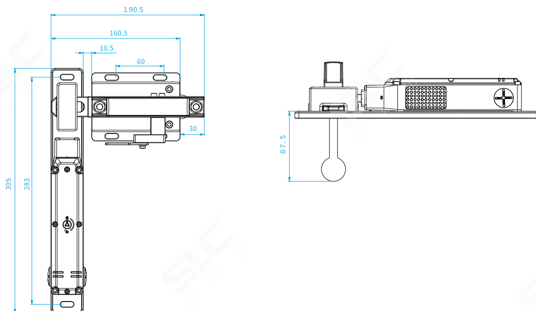
TSL4配TRL1系列安全联锁安装图
