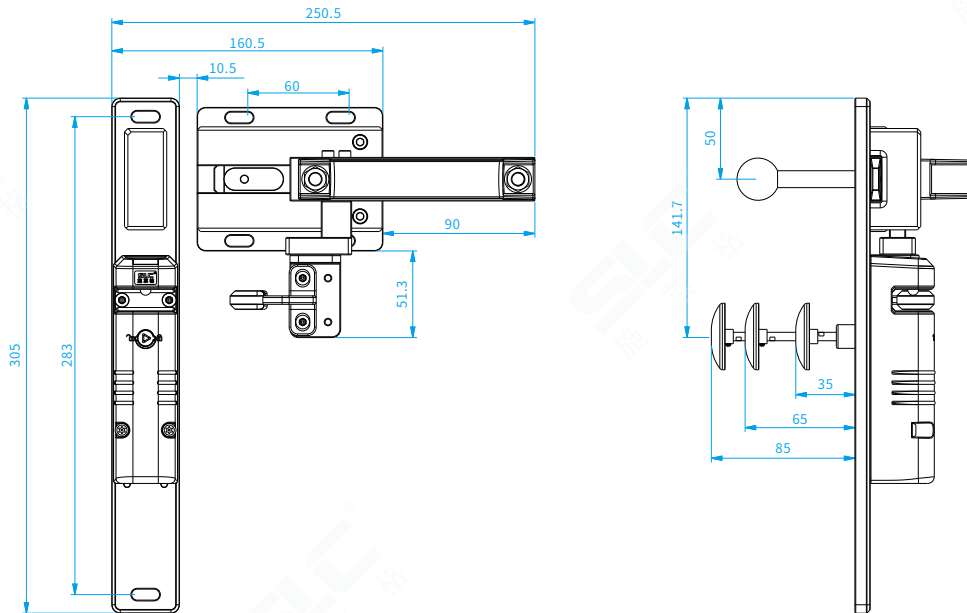
TSL4配TBL系列安全联锁安装尺寸
