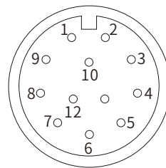
线缆母头
