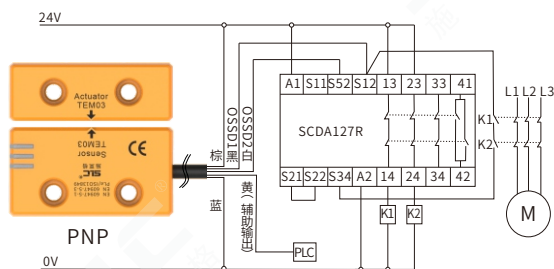
TEM02DPU安全开关PNP型输出接线示例
