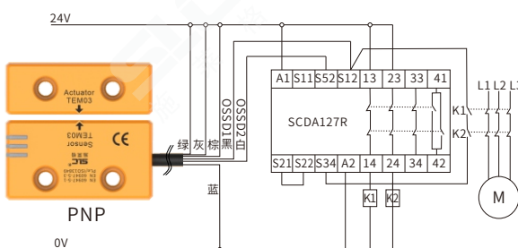
TEM03CPU安全开关级联PNP型输出接线示例
