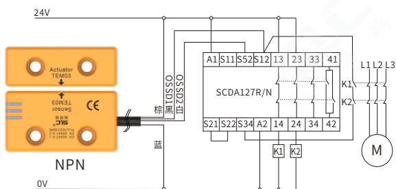
TEM03DN安全开关NPN型输出应用接线示例
