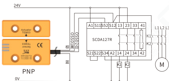
TEM03DP安全开关PNP型输出接线示例
