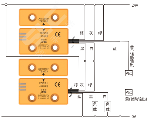
TEM03CPU安全开关级联PNP型输出级联接线示例
