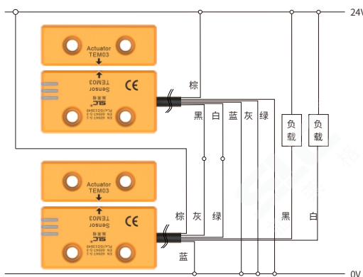
TEM03CN安全开关级联NPN型输出级联接线示例
