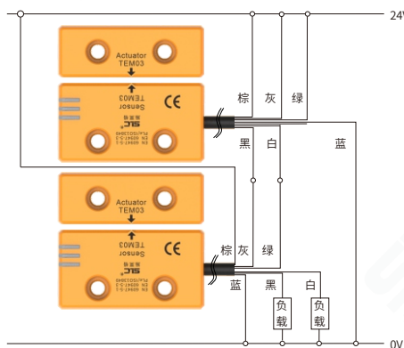
TEM03CP安全开关级联PNP型输出级联接线示例
