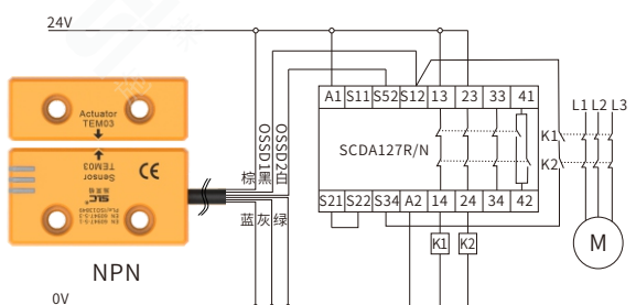
TEM03CNU安全开关级联NPN型输出应用接线示例
