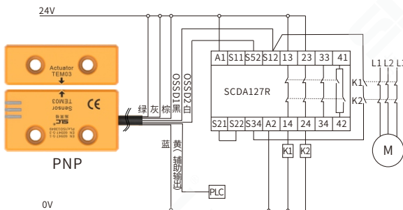
TEM03CPU安全开关级联PNP型输出接线示例
