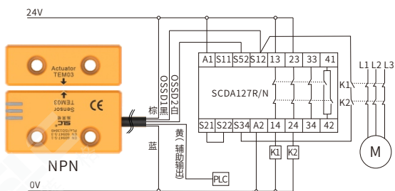
TEM02DNU安全开关NPN型输出应用接线示例
