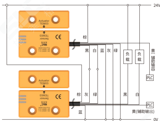
TEM03CNU安全开关级联NPN型输出级联接线示例
