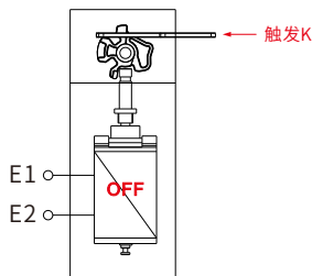
插入钥匙，电磁铁未通电
