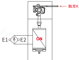
插入钥匙，电磁铁通电
