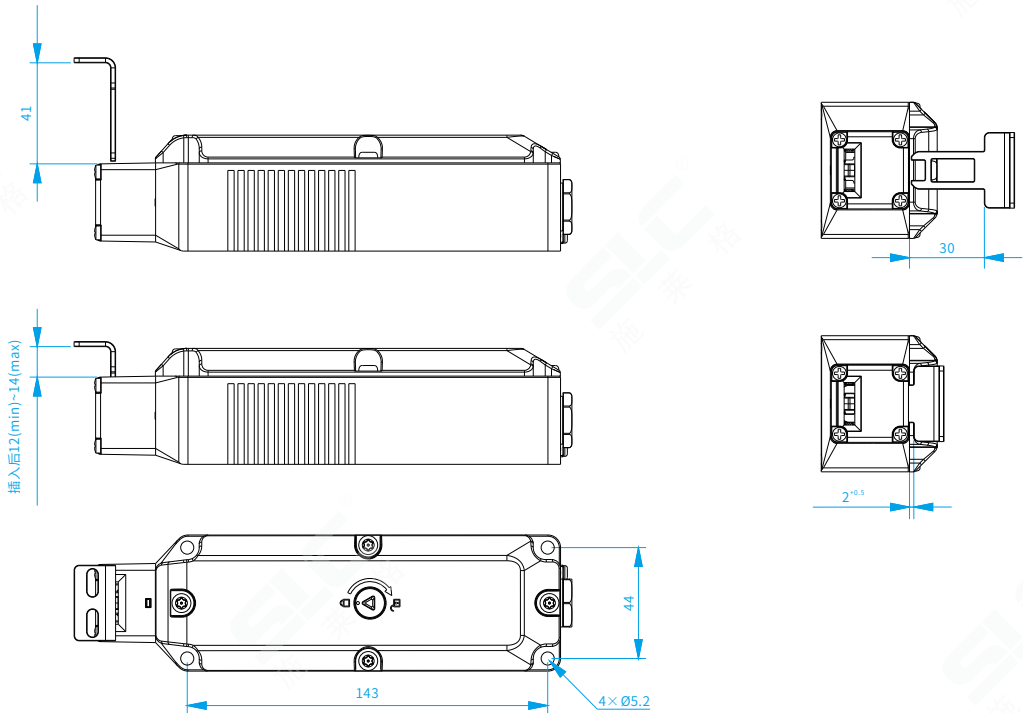
弯钥匙插入尺寸
