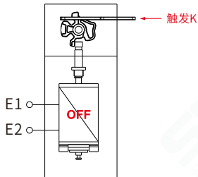
插入钥匙，电磁铁未通电
