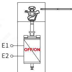
钥匙未插入或拔出钥匙后
