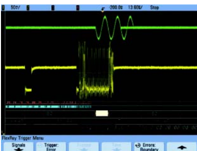
用MSO在FlexRay系统中进行混合信号测量
