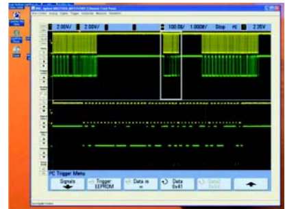
在网络浏览器中运行的 Agilent 远地前面板
