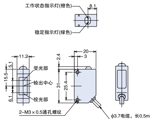
CX-462 传感器
