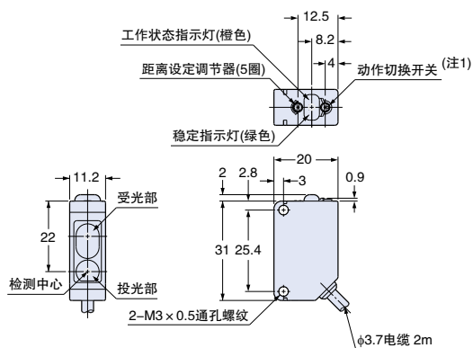
CX-44□ 传感器
