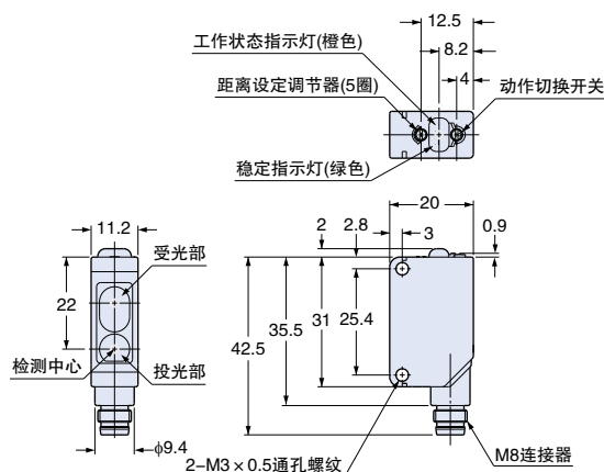
CX-44□-Z 传感器
