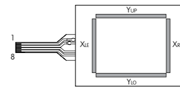
XLE, XRI: 上部电极端子 YUP, YLO: 下部电极端子
