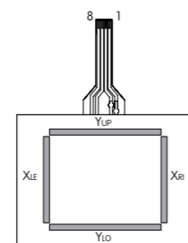
X1E, X1R: 上部电极端子 Y1U, Y1L: 下部电极端子
