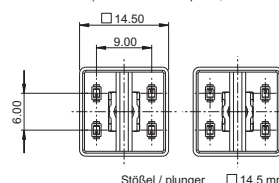
Stößel / plunger □ 14,5 mm
