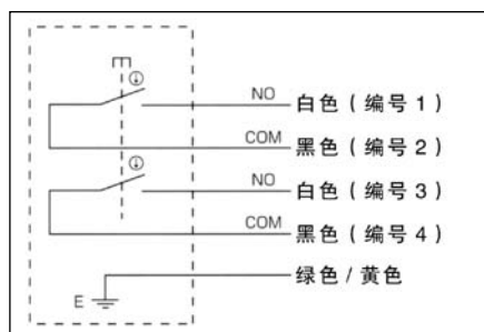
2TP用 连线图
