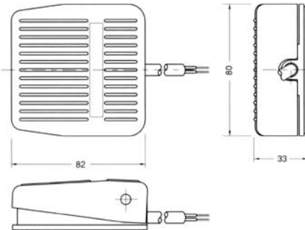
●外形尺寸为SFKB-1型号
