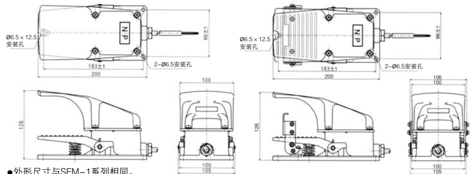
●外形尺寸与SFM-1系列相同。
