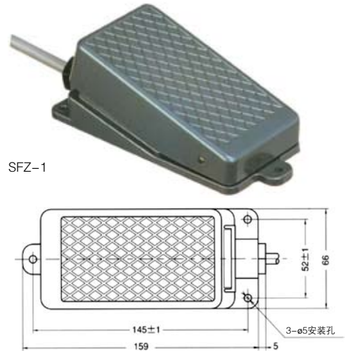
●外形尺寸SFZ系列相同。仅SFZ-1H全高64
