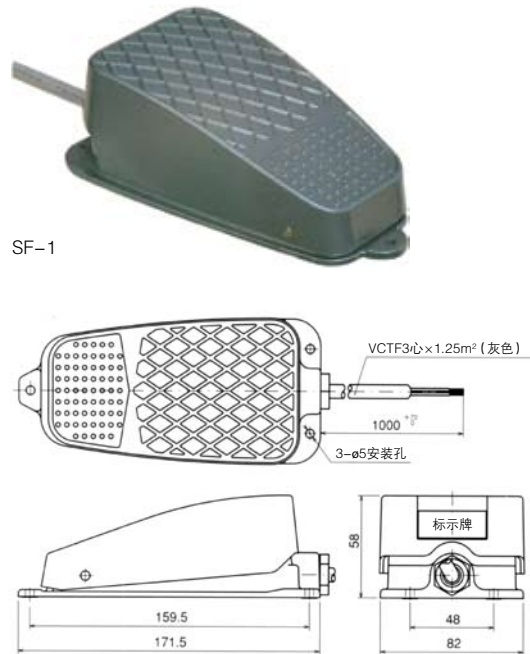
●外形尺寸SF系列相同。仅SF-1H·SF-1HN全高63
