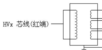
图 10 CT 接法
