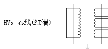
图7 PT接法
