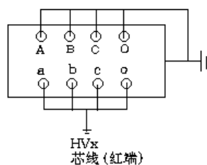
图 13 变压器接法
