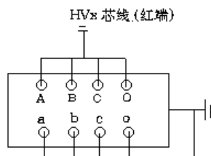
图 13 变压器接法
