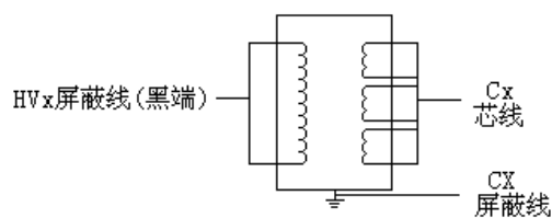
图 9CT 接法
