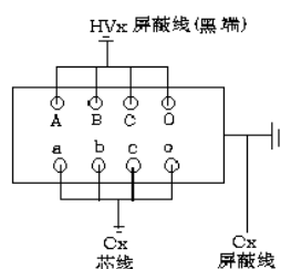
图 12 变压器接法
