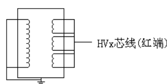
图8 PT接法
