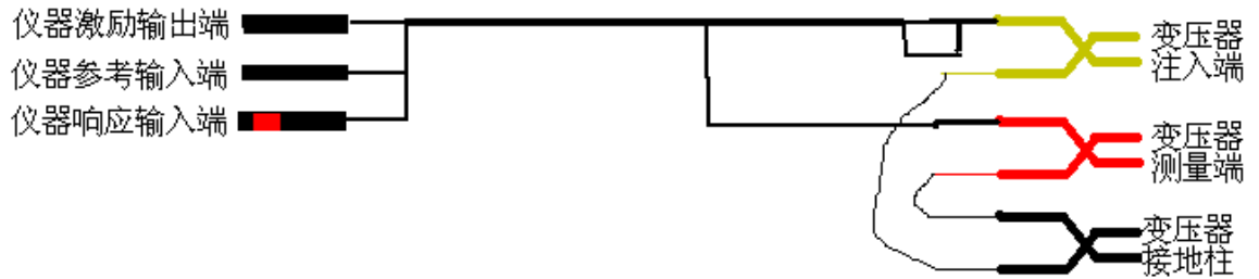
图 20 测试线连接示意图
