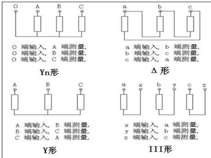
图 21 变压器 4 种常见接线方式
