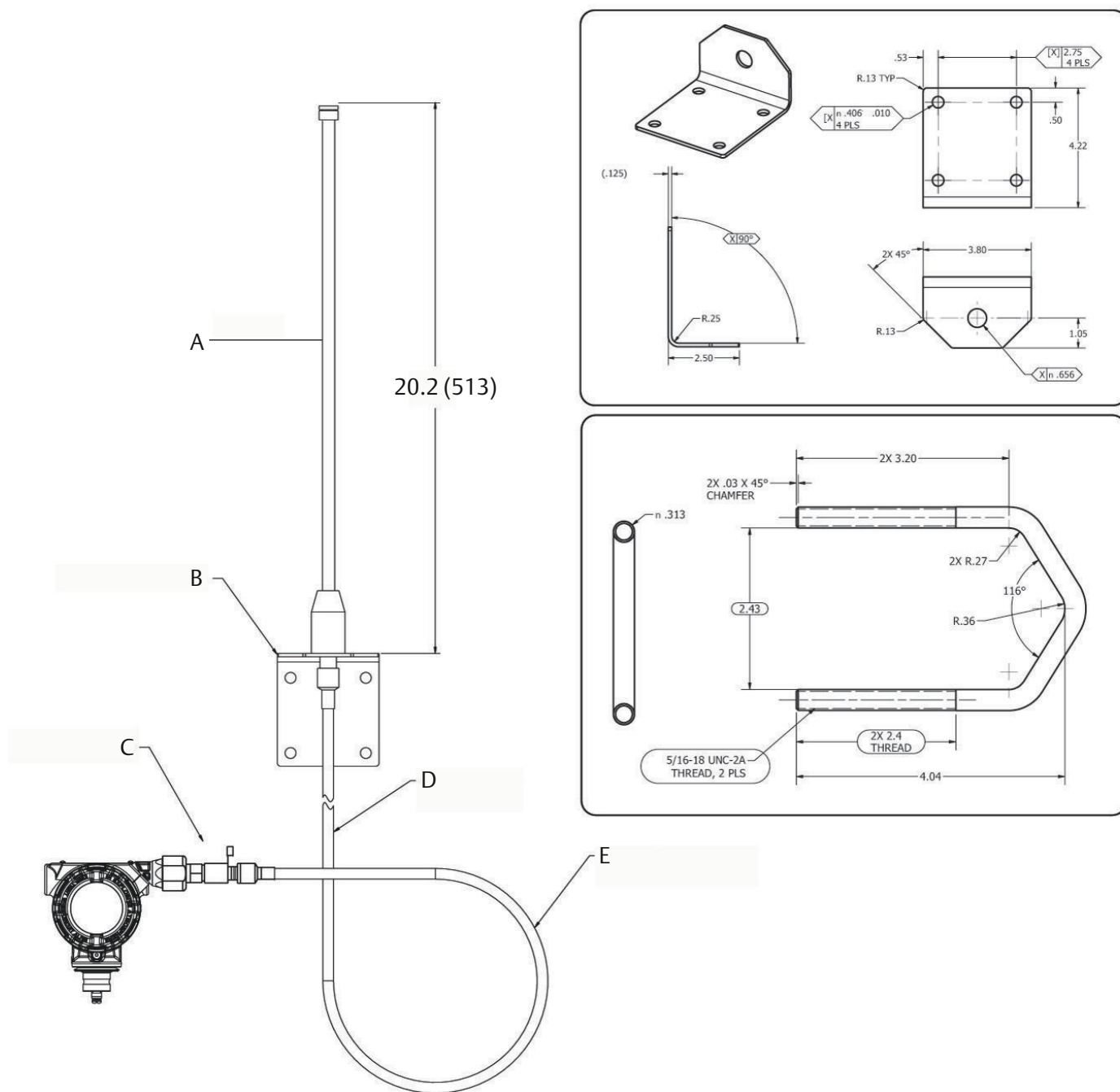
图 11: 高增益分体式天线 (WN 选项) :
