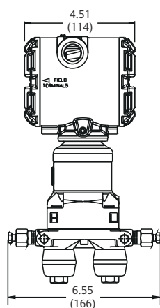
图 5: 带共平面传感器模块和法兰的变送器 (侧视图)
