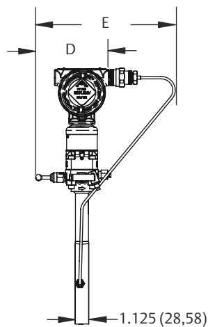
图 18: Rosemount 3051SFC 紧凑型孔板流量计 (代码为 C 和 P 的一次元件类型)
