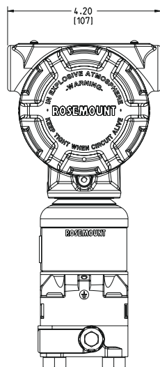
图 4: 带共平面传感器模块和法兰的变送器 (前视图)
