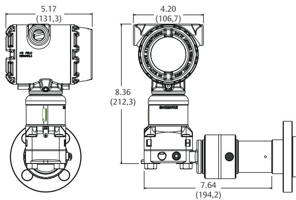
图 26: Rosemount 3051S 可扩展液位变送器，带宽温变送器
