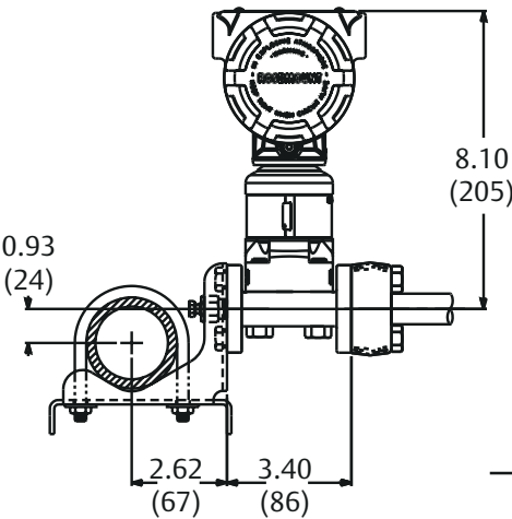
图 13: 传统安装组态
