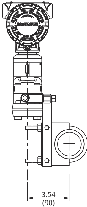
图 12: 共平面安装组态 ( B4 支架 )
