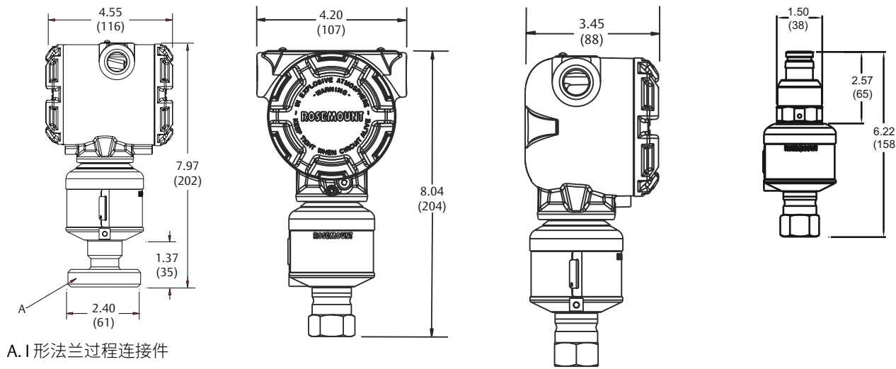
图 10: Plantweb 外壳、接线盒外壳以及快速连接直连式 SuperModule™ 平台
