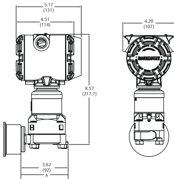
图 25: Rosemount 3051S 可扩展液位变送器，带 SC 密封件
