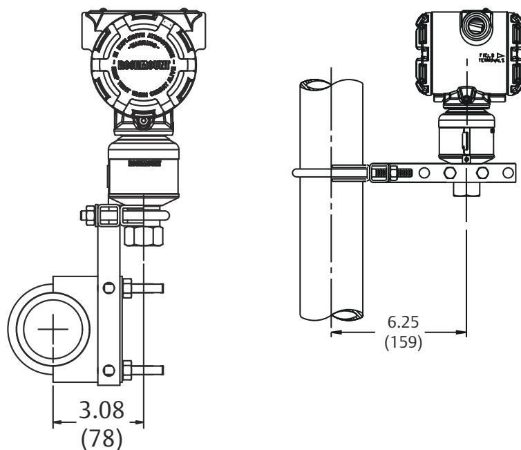
图 14: 直连式安装组态 (B4 支架)
