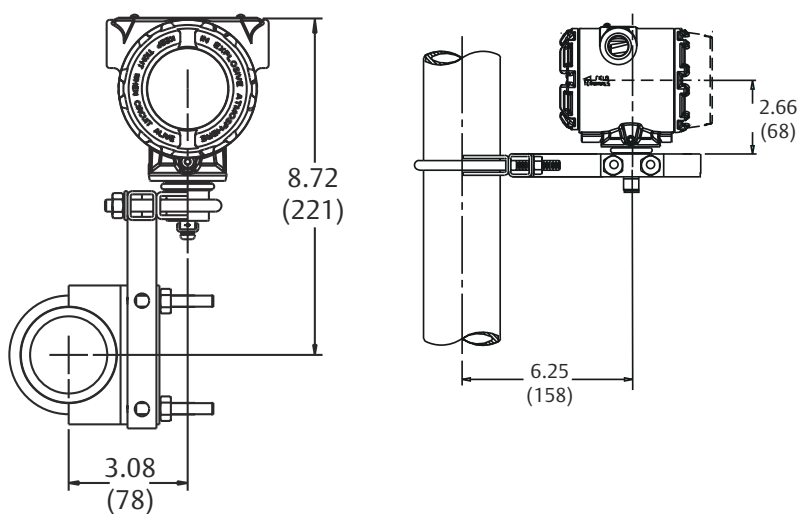
图 15: 分体式显示器安装组态 (B4 支架)
