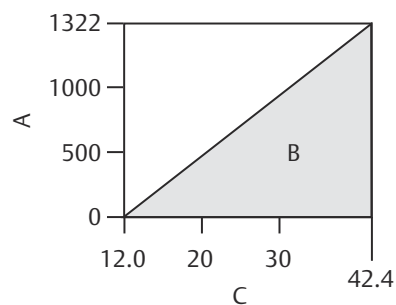
图 2: 带 HART 诊断功能 (选项代码 DA2) 的 Rosemount 3051SMV 和 3051SF_1-7、3051S 和 3051SF_D
