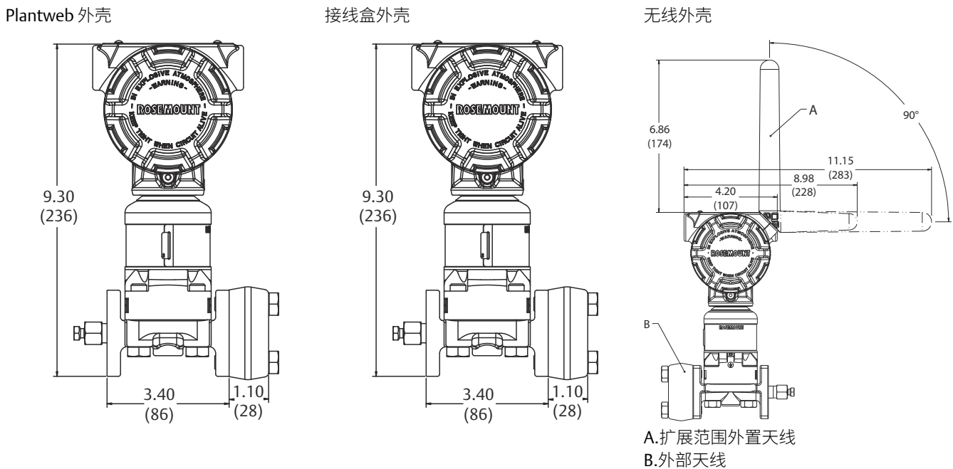
图 6: 带共平面传感器模块和传统法兰的变送器 (前视图)
