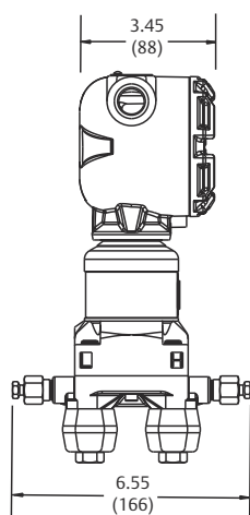
图 5: 带共平面传感器模块和法兰的变送器 (侧视图)
