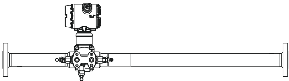
图 19: 罗斯蒙特 3051SFP 一体化孔板流量计
