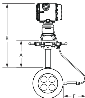
图 18: Rosemount 3051SFC 紧凑型孔板流量计 (代码为 C 和 P 的一次元件类型)
