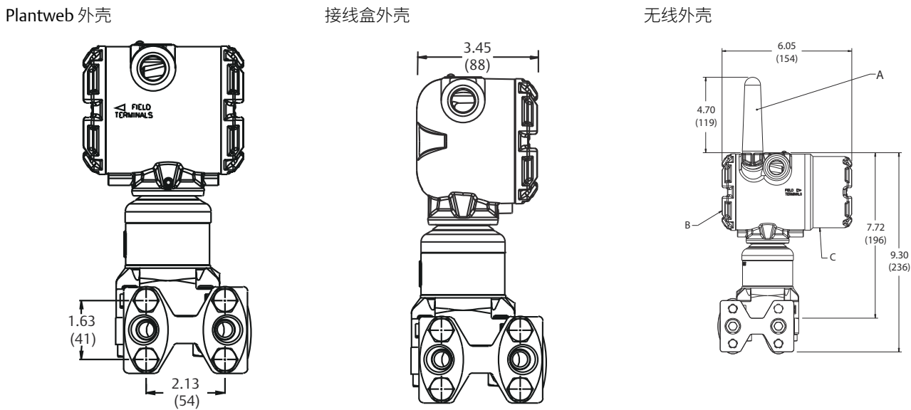
图 7: 带共平面传感器模块和传统法兰的变送器 (侧视图)
