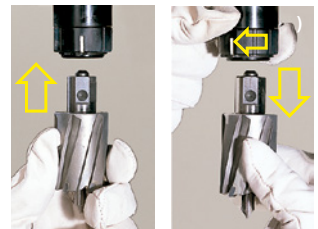
刀具安装 / 刃物の取り付け 刀具卸载 / 刃物の取り外し
