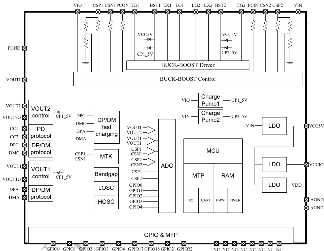
图 3 IP6559 内部框图
