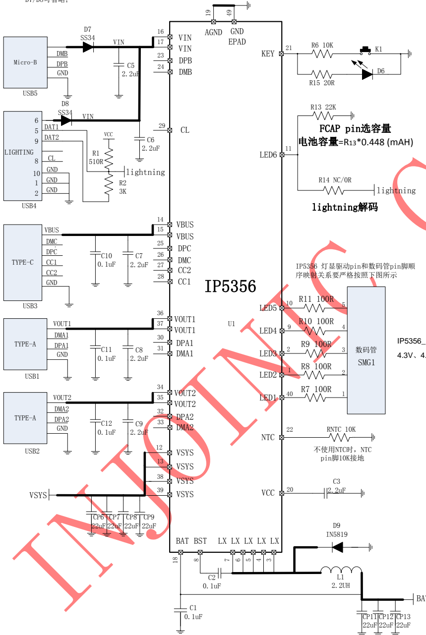
图 21 IP5356_188 系列应用的典型应用原理图
