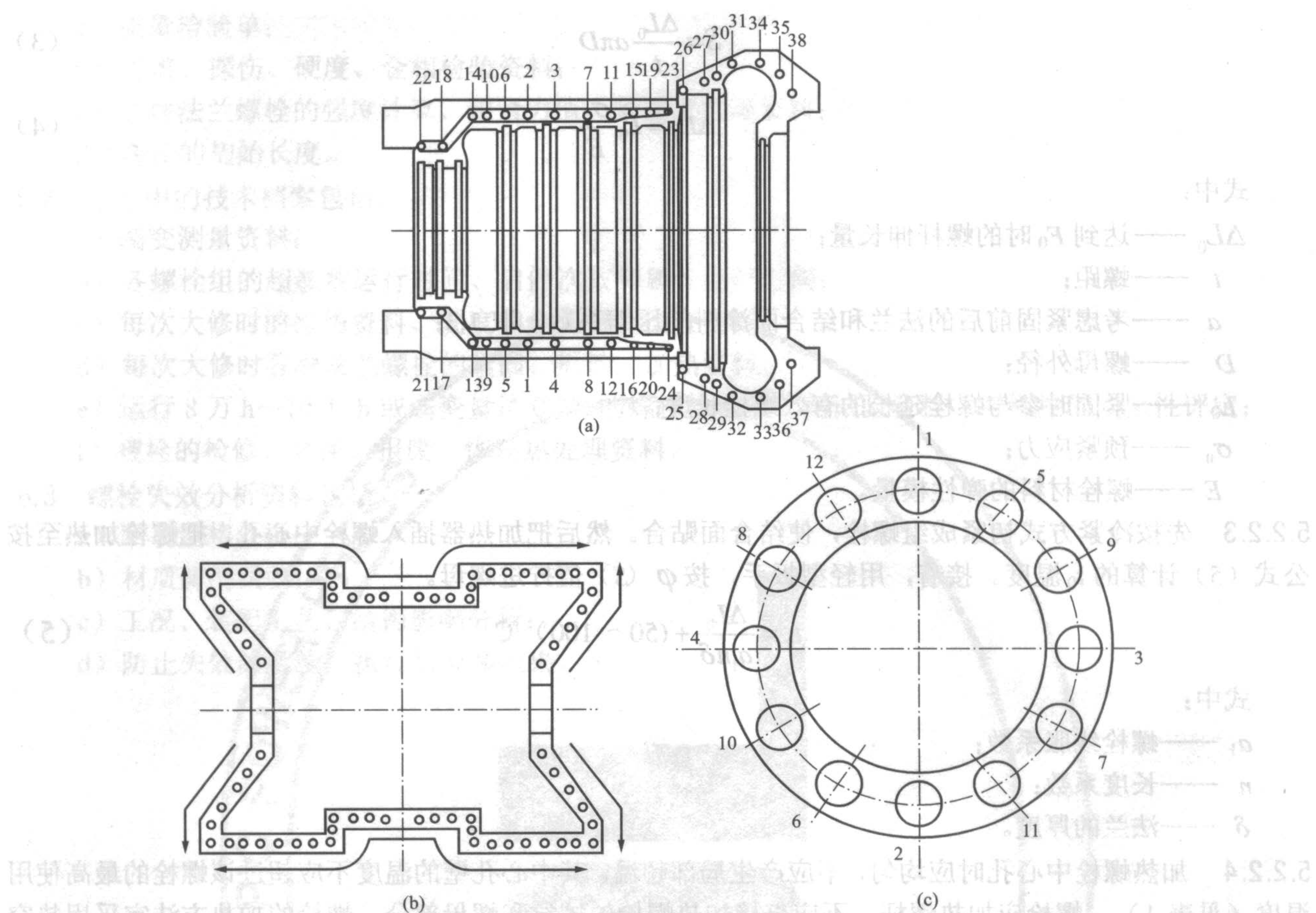
(a) 高压缸法兰；(b) 双排汽低压缸法兰；(c) 阀门圆法兰
