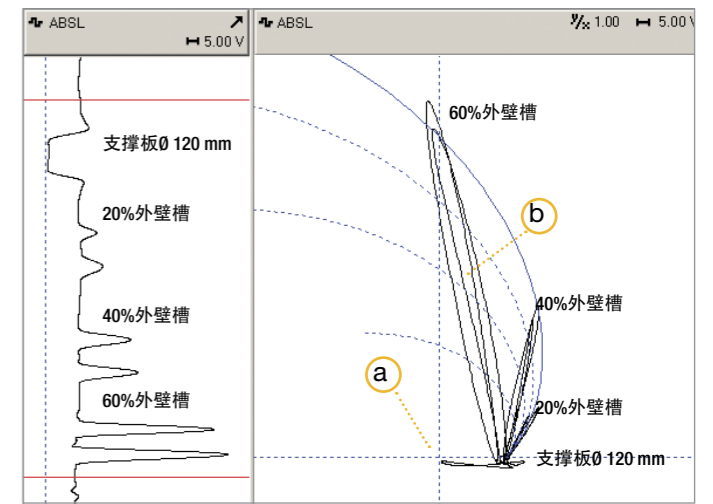
a) 支撑板信号的“原始偏移”已被减到最小，以更快地完成RFT校准。 b) 现在，单励磁器探头模式中的拾波器和励磁器的效果信号极为相似。
