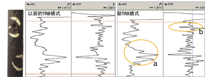
a) 经过优化的新型线圈可更好地区分内壁凹坑的缺陷指示 b) 新型设计可使出现在其它信号指示之间的通壁孔信号显得更清晰
