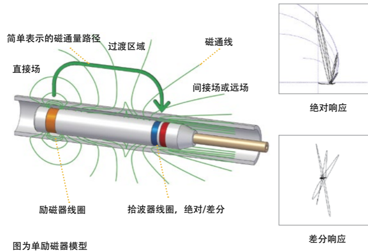
图为单励磁器模型
