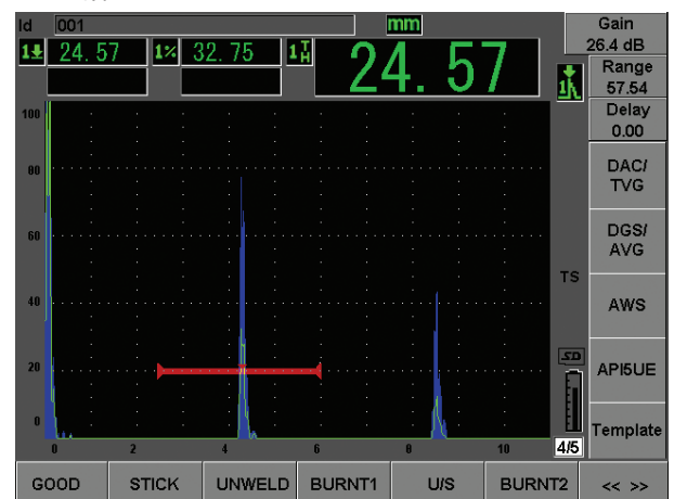
EPOCH 600型仪器的动态DAC/TVG特性
