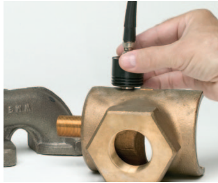
35HP测厚仪可以测量汽缸内腔和许多其它金属铸件以及具有声速衰减性的材料。
