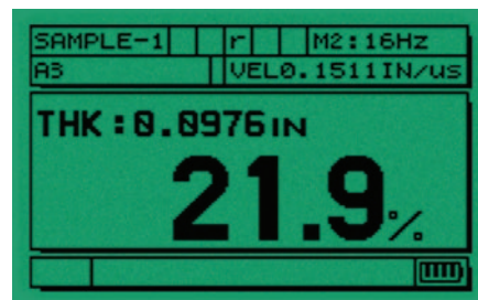
材料减薄程度以百分比表示。
