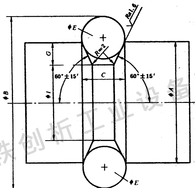
图 B.2 心轴
