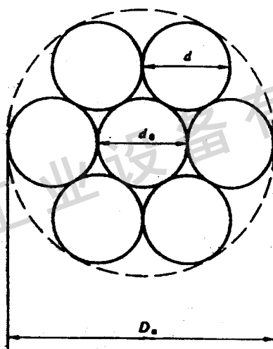
图3 1×7结构钢绞线外形示意图
