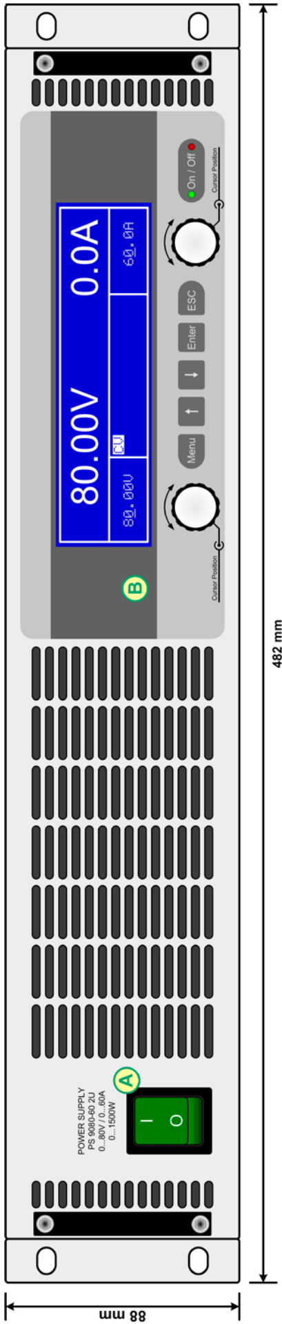
图 1 - 前视图
