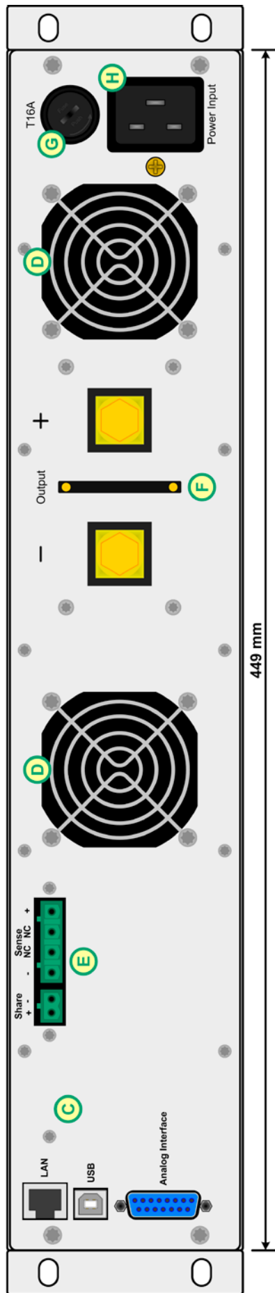
图 2 - 后视图
