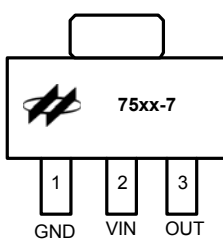
SOT89-3
