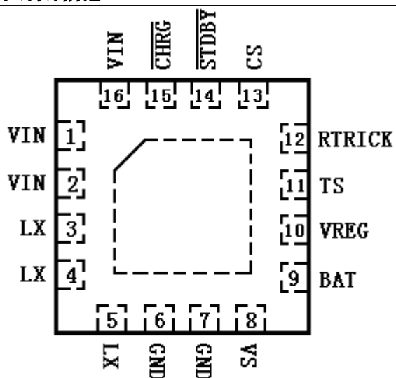
16 引脚 4mm*4mmQFN16 封装顶视图 (散热片接地不可接其他电位)
