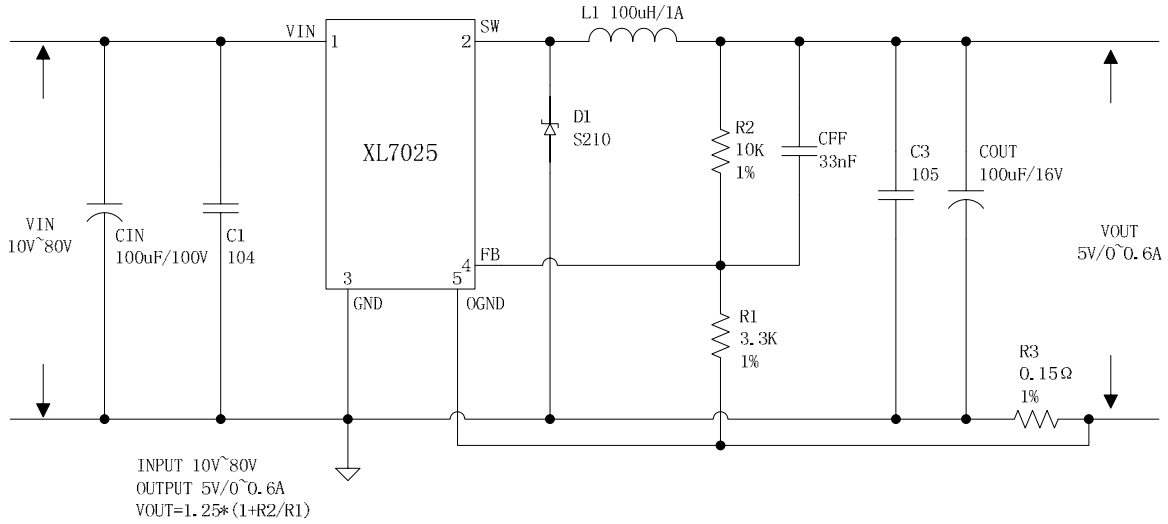
图 9. XL7025 系统参数测量电路(VIN=10V~80V, VOUT=5V/0.6A)
