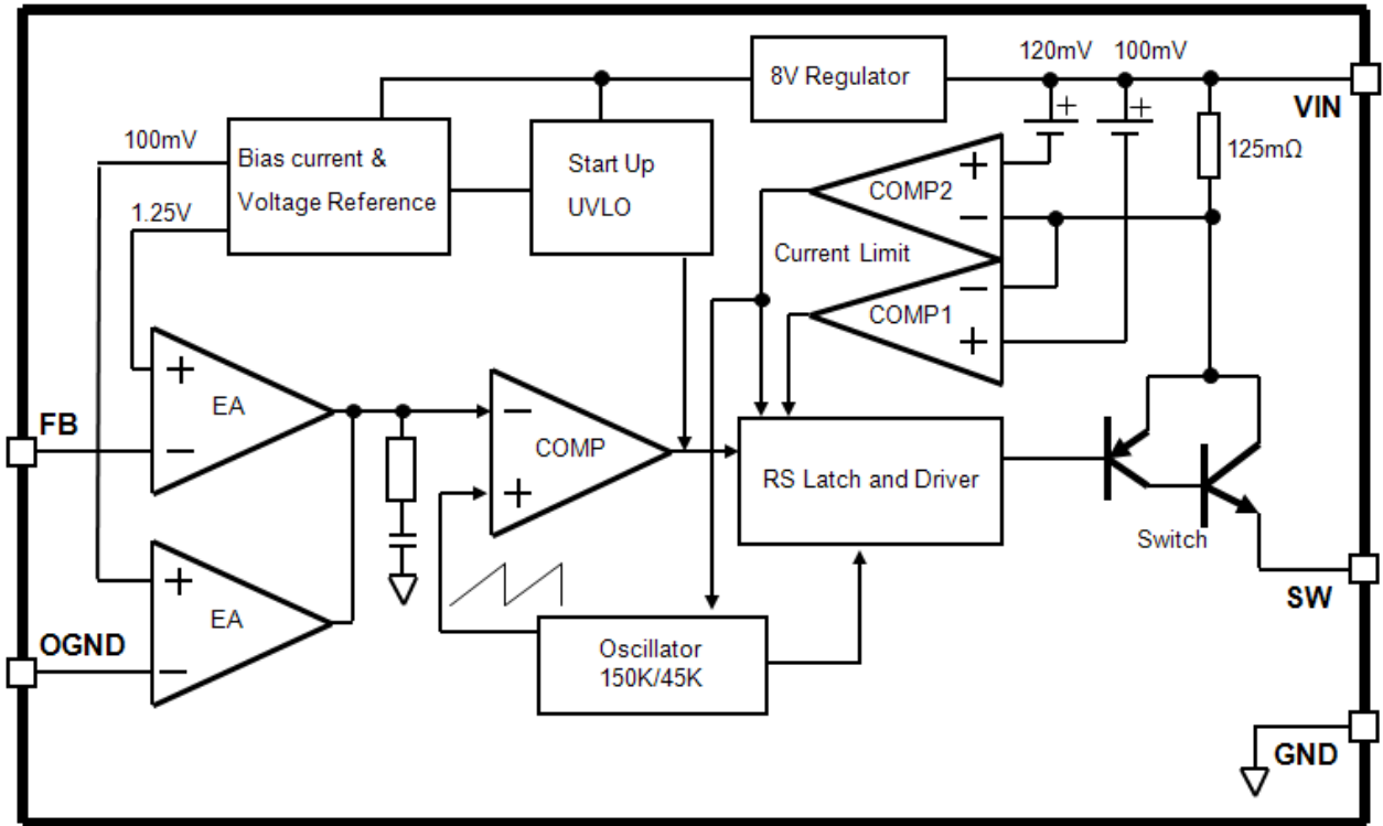
图 3. XL7025 方框图
