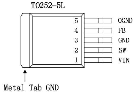
图 2. XL7025 引脚配置
