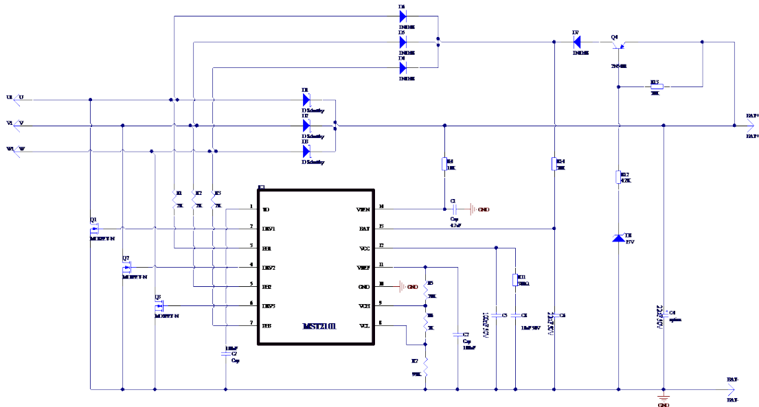
三相磁电机调压器应用图
