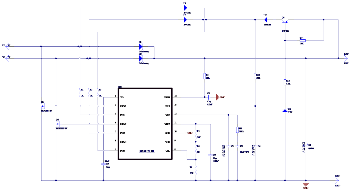
单相磁电机调压器应用图
