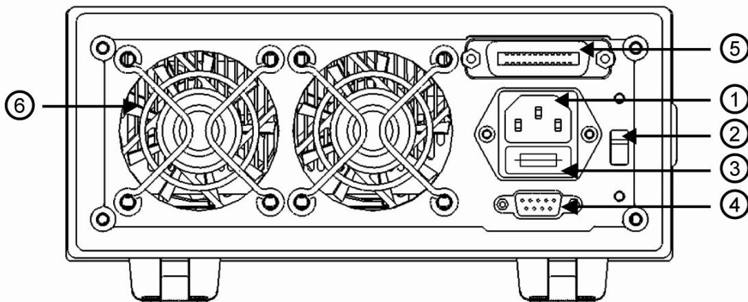
图 1-2 后面板图
