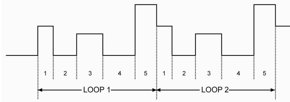
图 2-9 序列测试
