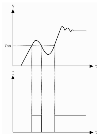
图 2-12 启动电压锁定(Von Latch)关闭
