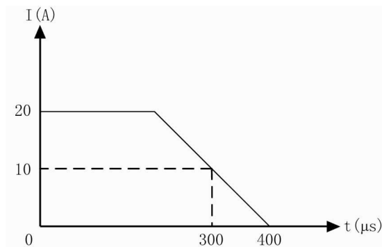
图 2-15 电流下降速率示意图
