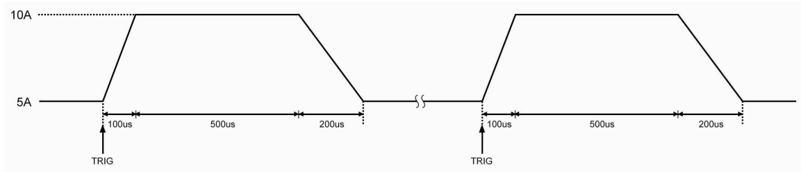
图 2-7 脉冲方式
