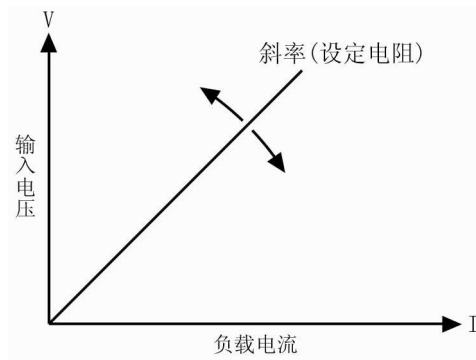
图 2-3 定电阻模式
