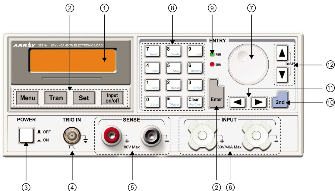
图 1-1 前面板图
