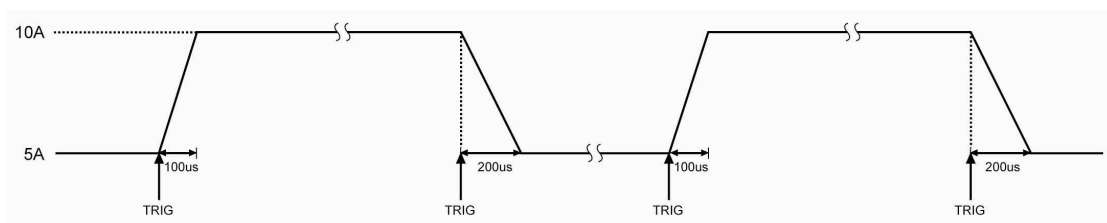
图 2-8 翻转方式
