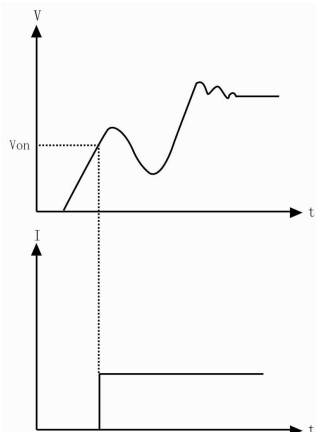
图 2-11 启动电压锁定(Von Latch)打开
