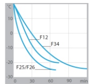
制冷曲线 溶液：乙醇
