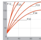
加热曲线： 溶液：Thermal浴油
