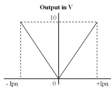
(图3：0-10VDC 输出)
