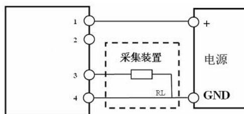
电压型输出接线示意图
