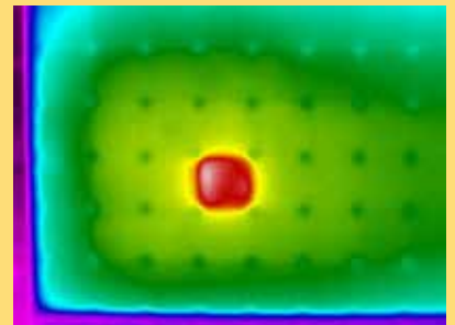
检测太阳能电池板热斑，发现工艺和质量问题
