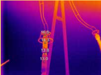
避雷器阀片受潮或老化
