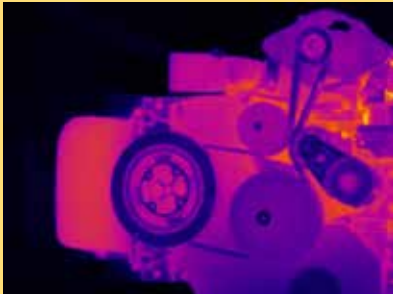
对发动机的散热系统、排气系统、传动系统进行热分布检测，改善设计布局
