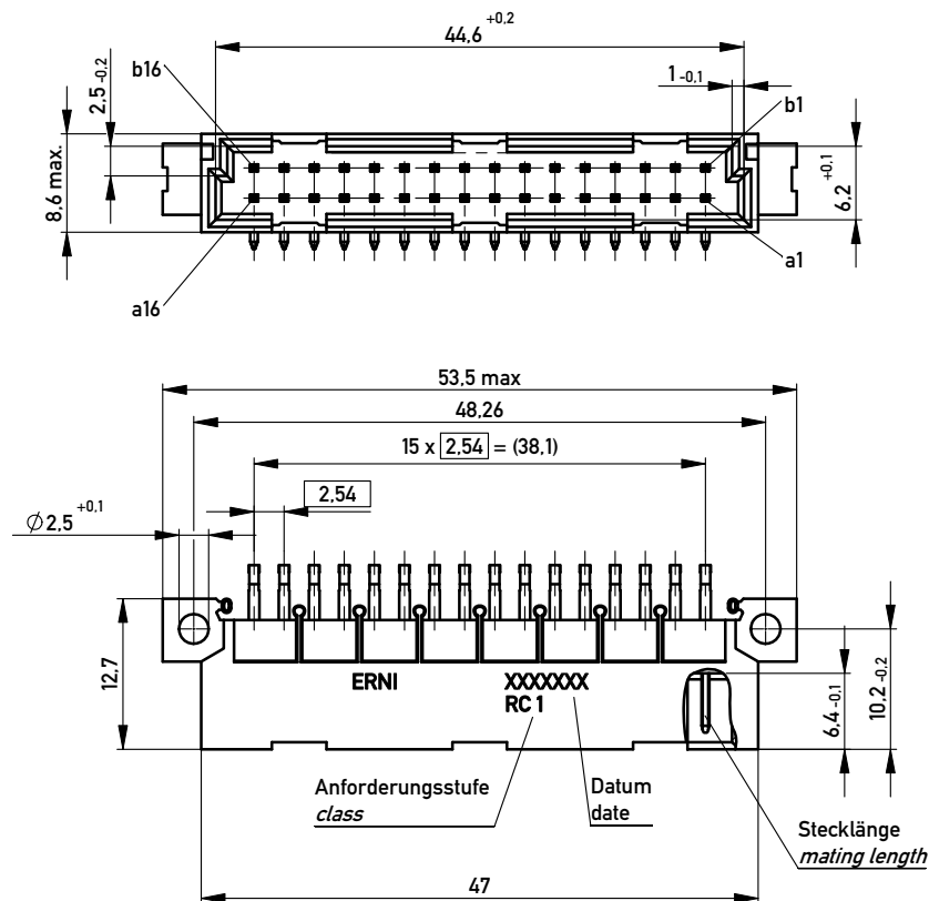
Bestückungsplan / contact layout
