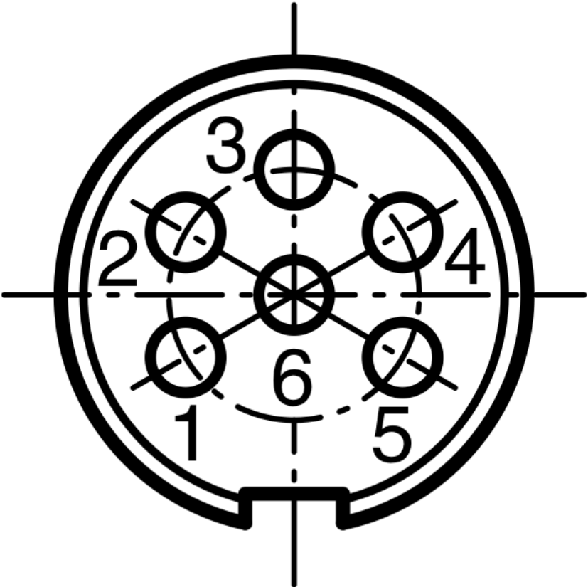
Kontaktanordnung
