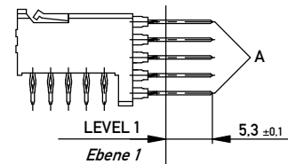
CONTACT LENGTH EXAMPLES Kontaktlänge Beispiele
