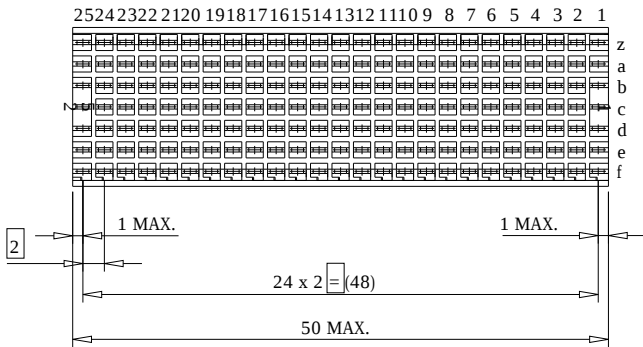
CONTACT LAYOUT BESTUECKUNGSPLAN
