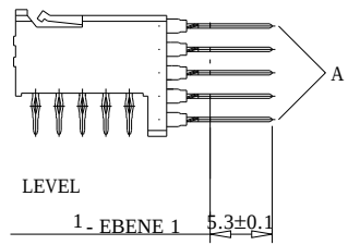
CONTACT LENGTH EXAMPLES KONTAKT LAENGE BEISPIELE
