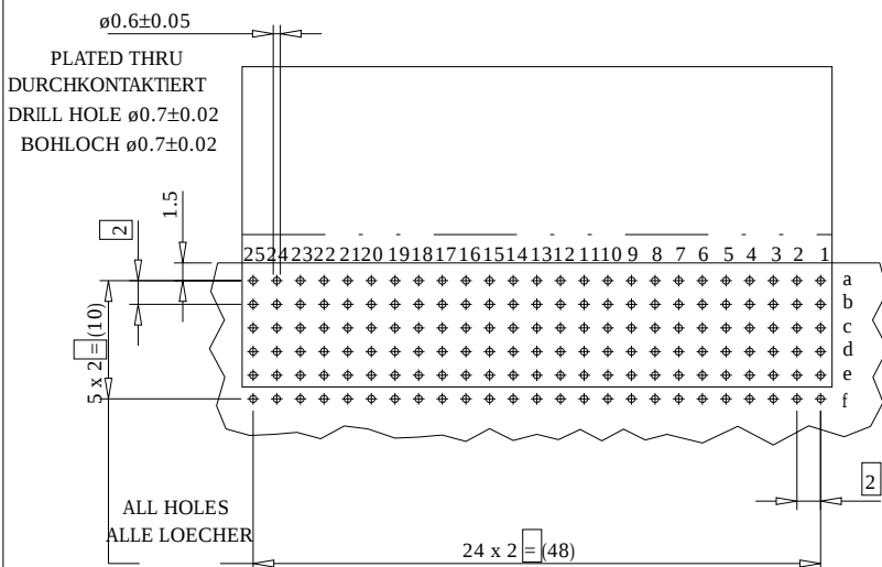
BOARD HOLE PATTERN (COMPONENT MOUNTING SIDE) LOCHBILD FUER LEITERPLATTE (BESTUECKUNGSSEITE)
