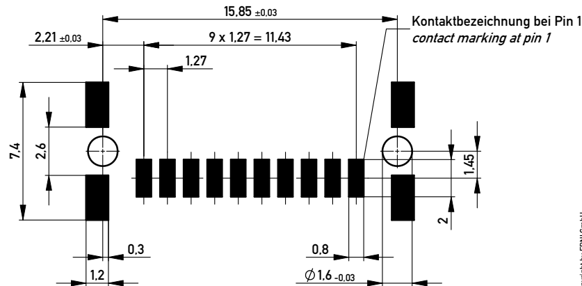
Leiterplatten-Layout für SMT PCB-Layout for SMT
