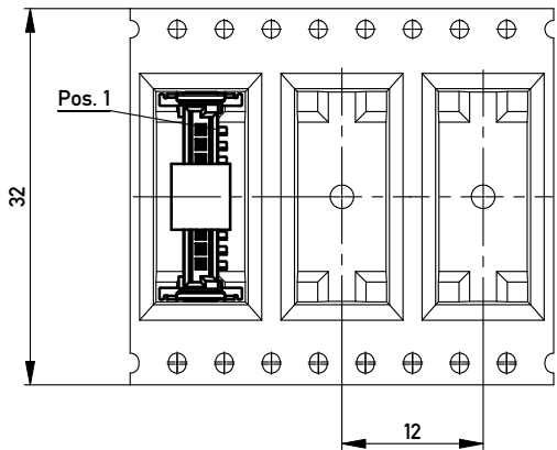
Abspulrichtung - Reel off Direction
