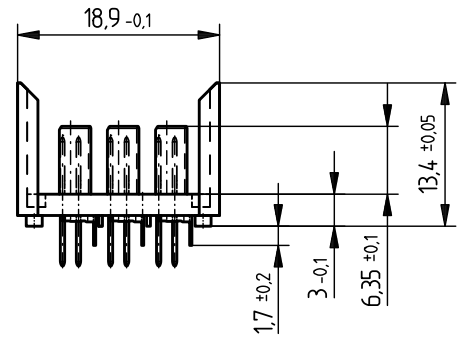
Kontaktversionen, Messerkontakte Contact Selection Options, Male Contacts
