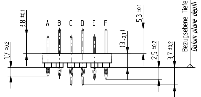
Kontaktversionen, Messerkontakte Contact Selection Options, Male Contacts
