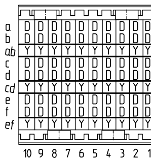
Bestückungsplan - contact layout
